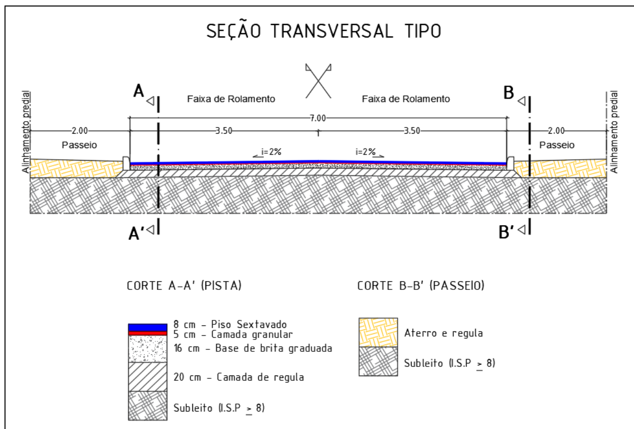
Imagem 3 - Seção tipo de pavimentação em tangente
