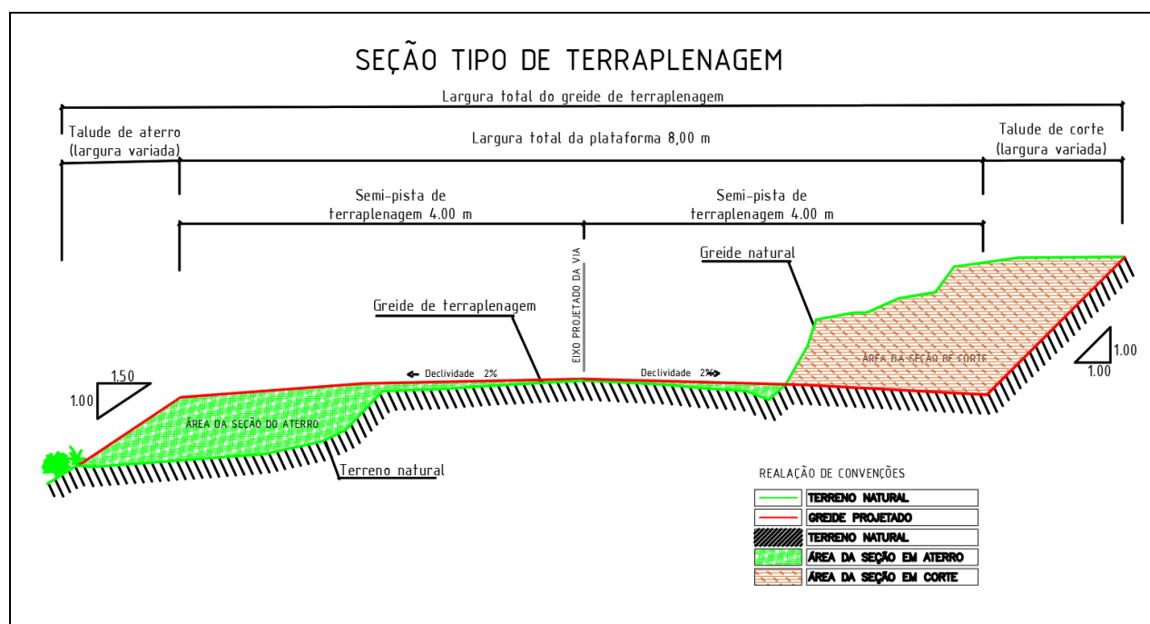
Imagem 4 - Seção tipo de terraplenagem em tangente
