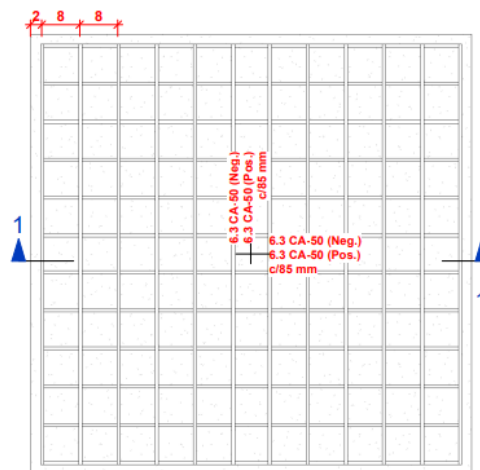
01 TAMPA DE CONCRETO ARMADO 1 : 10
