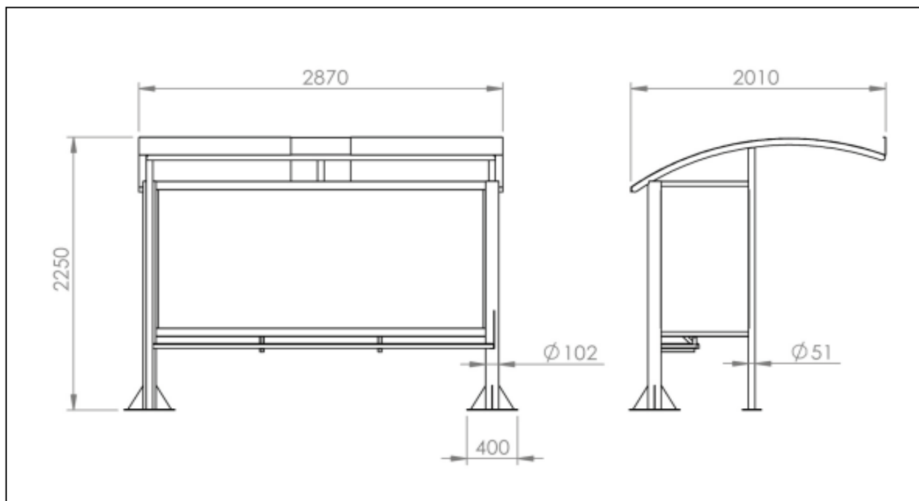
Figura 1: Detalhamento Técnico do Abrigo 01 – Modelo de Referência (Botuverá)
