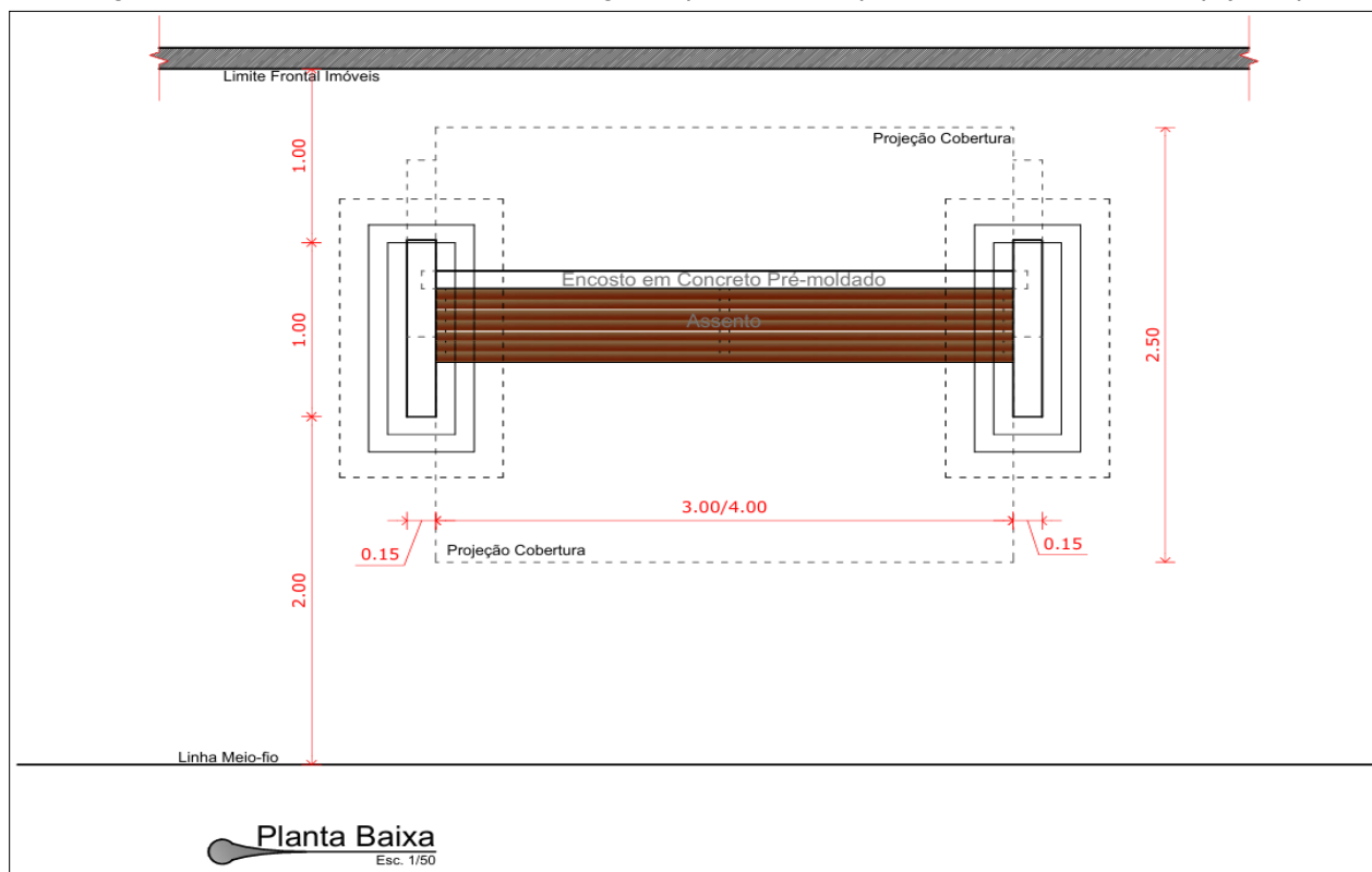
Figura 6: Detalhamento Técnico do Abrigo 02 (Planta Baixa) – Modelo de Referência (Tijucas)
