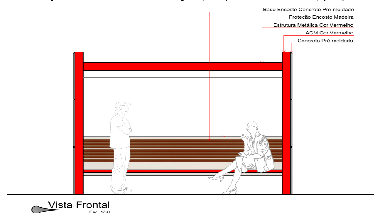
Figura 4: Detalhamento Técnico do Abrigo 02 (frontal) – Modelo de Referência (Tijucas)
