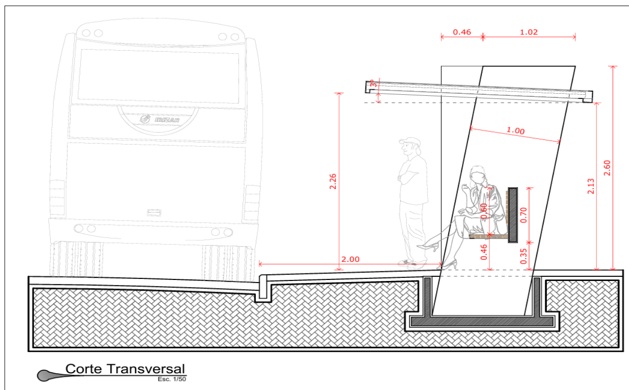
Figura 5: Detalhamento Técnico do Abrigo 02 (Transversal) – Modelo de Referência (Tijucas)
