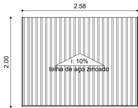
COBERTURA ESC.: 1/50
