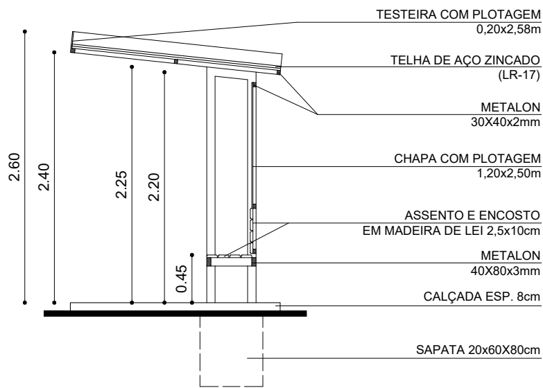
CORTE AA ESC.: 1/50
