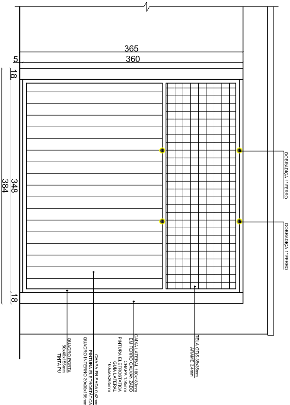
DETALHE PORTÃO 03 SEM ESCALA
