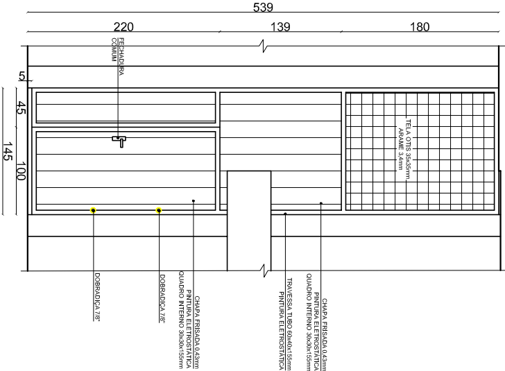
DETALHE PORTÃO 02 SEM ESCALA
