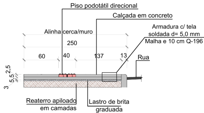
CORTE AA - PISO PASSEIO PADRÃO SEM ESCALA
