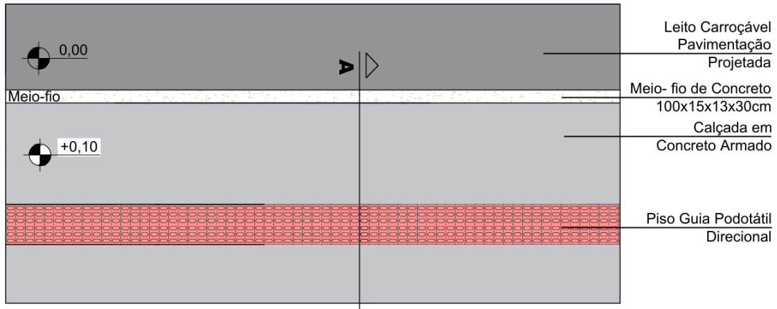
DETALHE - PISO PASSEIO PADRÃO SEM ESCALA
