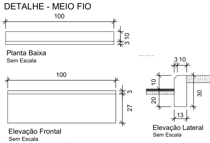
Figura 04 – Detalhamento Faixas de Uso Calçada Medindo 2,50m
