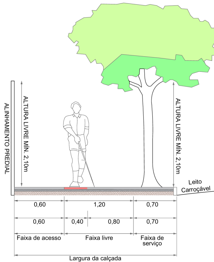
DETALHE FAIXAS DE USO CALÇADA MEDINDO 2,50 m Sem Escala
