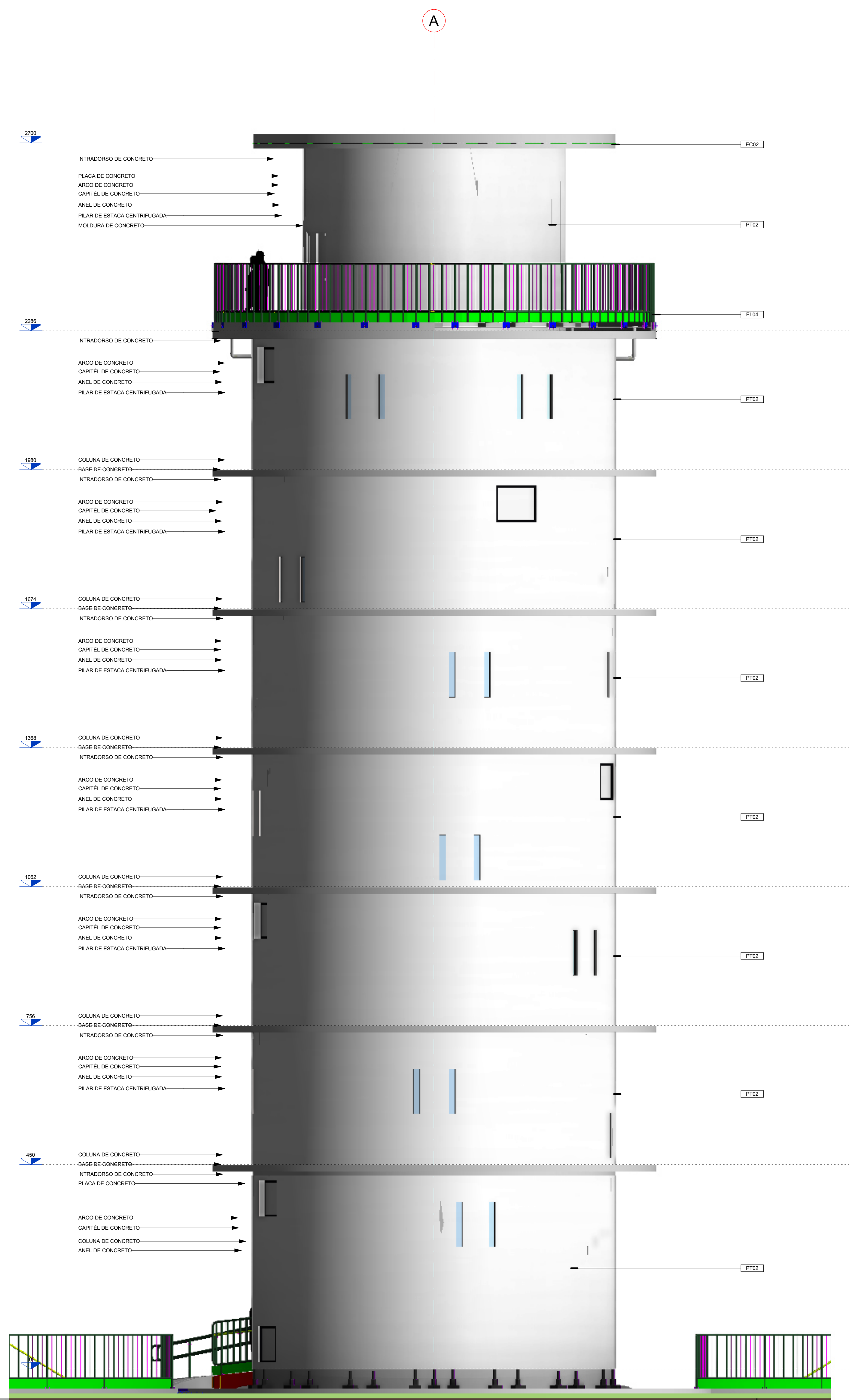
2 ELEVÇÃO LATERAL DIREITA ESCALA 1:50
