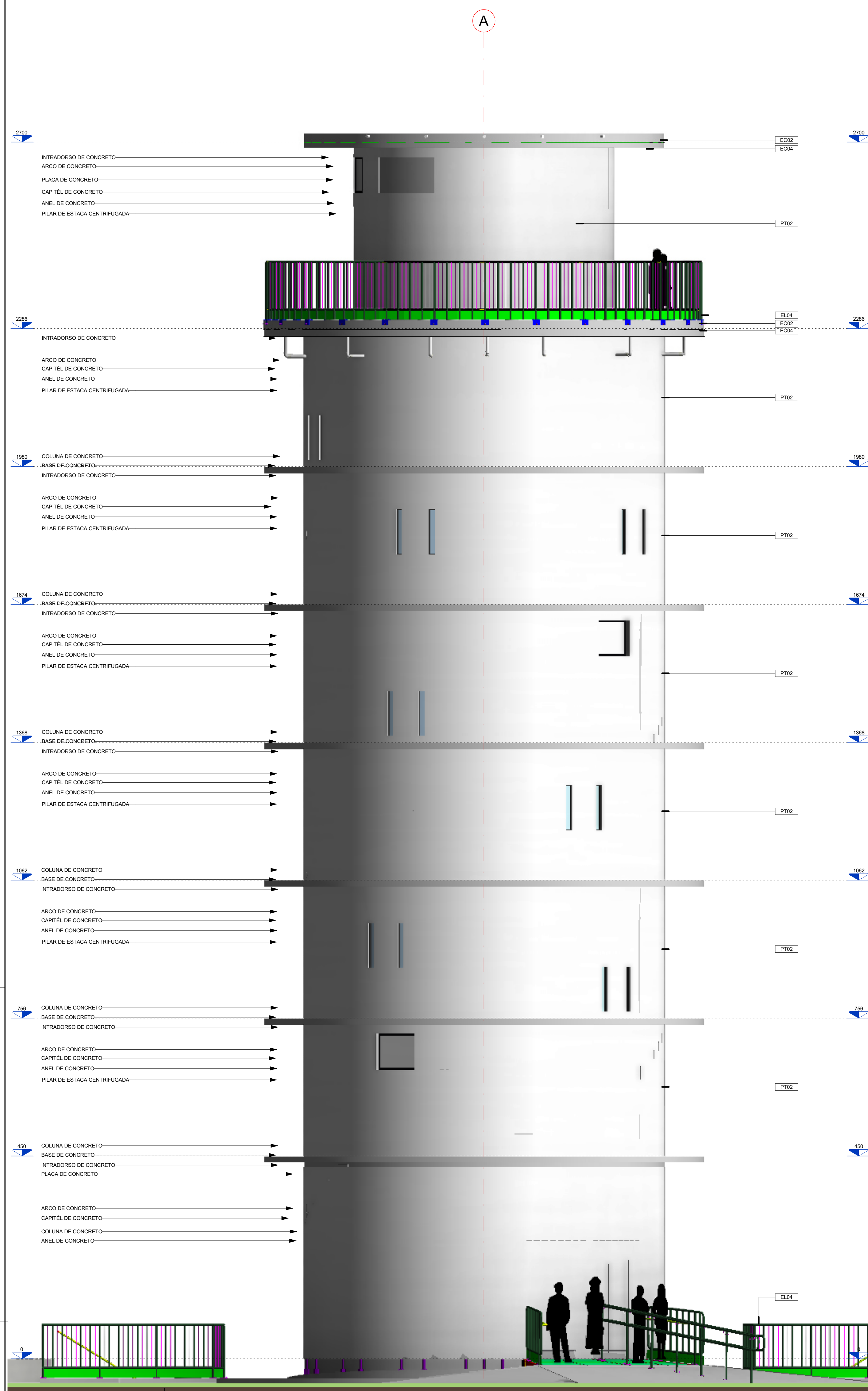
1 ELEVACÃO LATERAL ESQUERDA ESCALA 1:50
