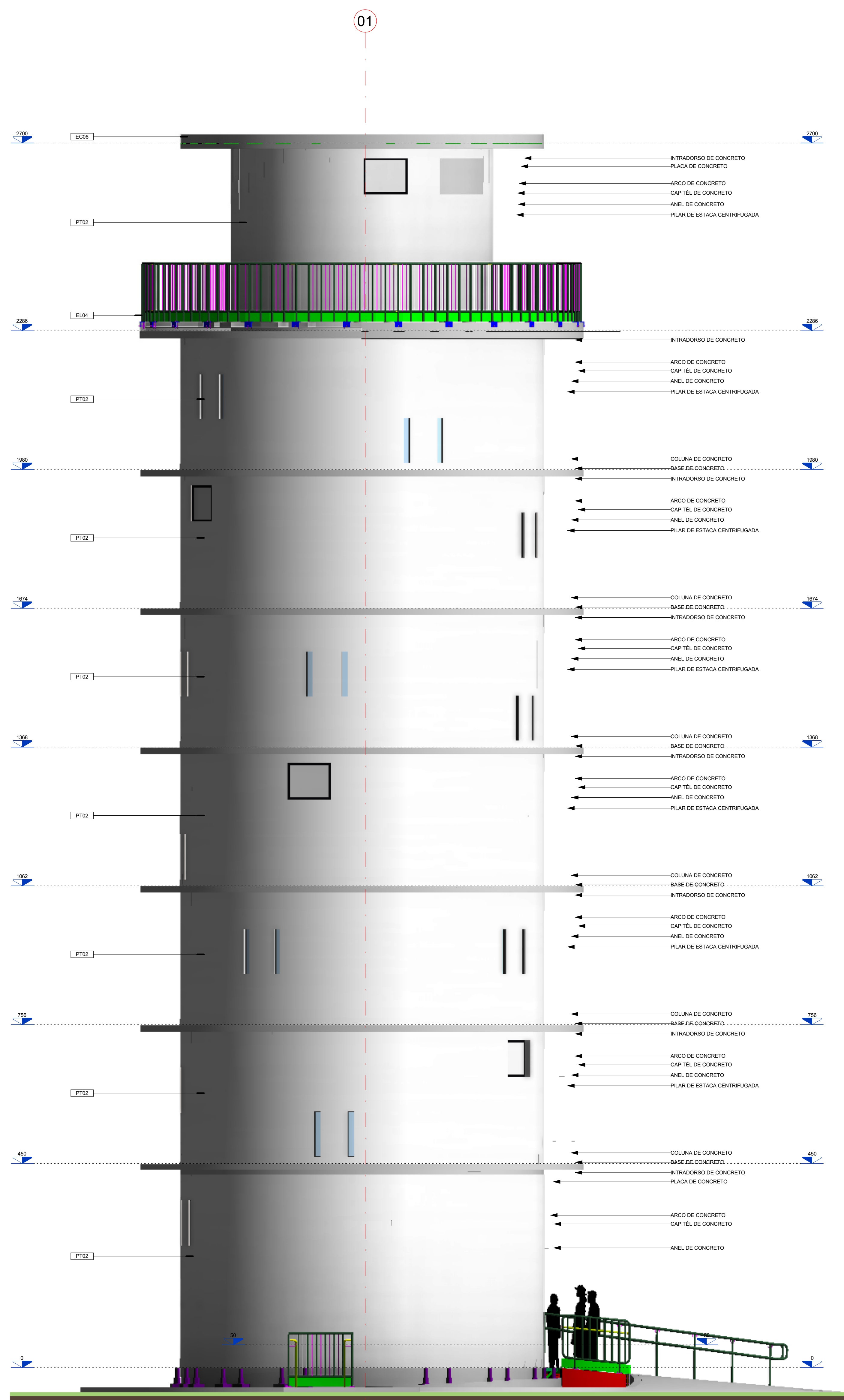
2 ELEVACÃO POSTERIOR ESCALA 1:50
