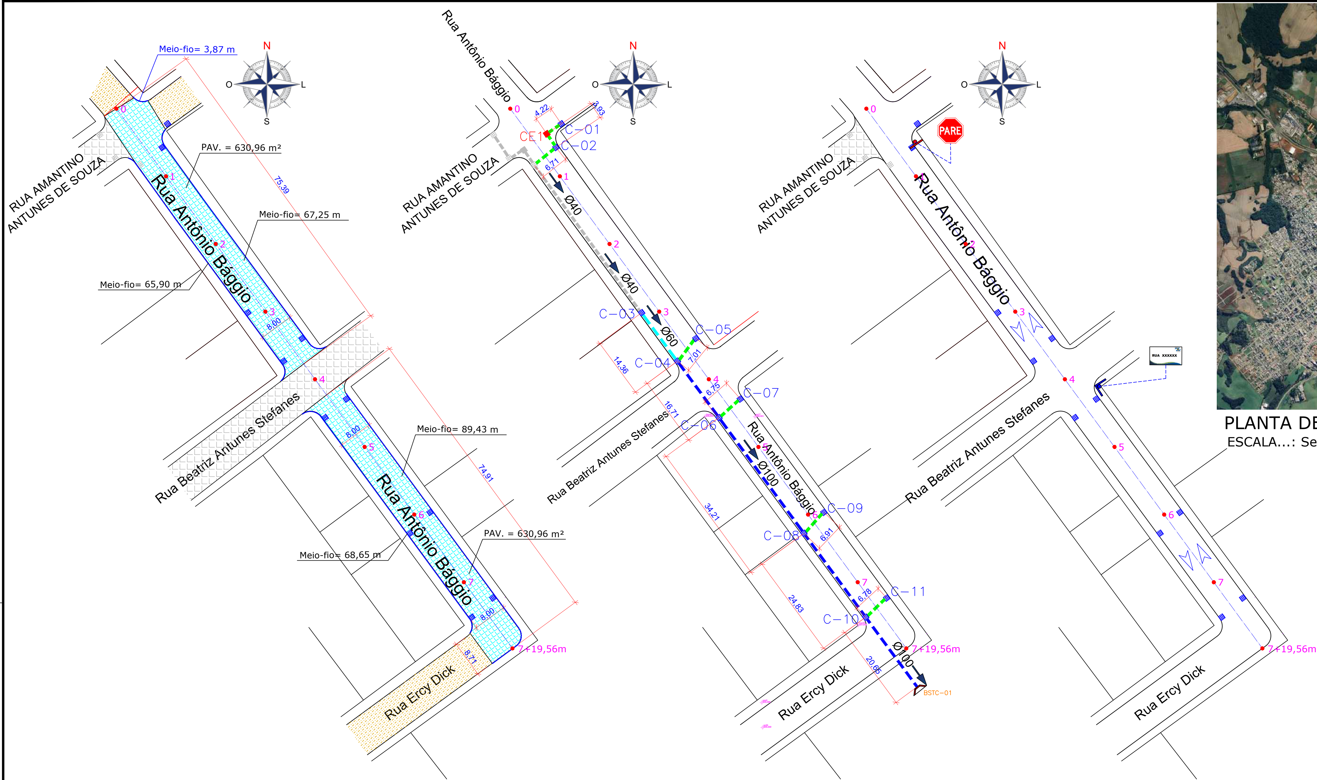
DRENAGEM ESCALA...: 1:500
