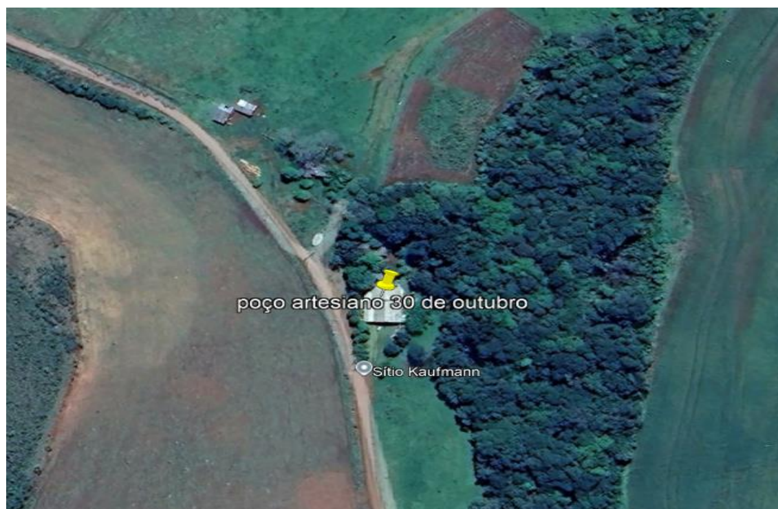
Planta de Situação –projeto do poço . Coord. UTM- 464285/6975532 -
