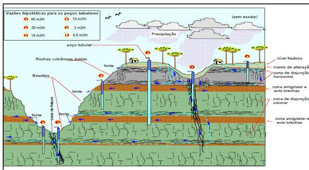
Fig. 3– Modelos de perfis regionais do Aquífero Serra Geral. Bacia Hidrográfica da Área
