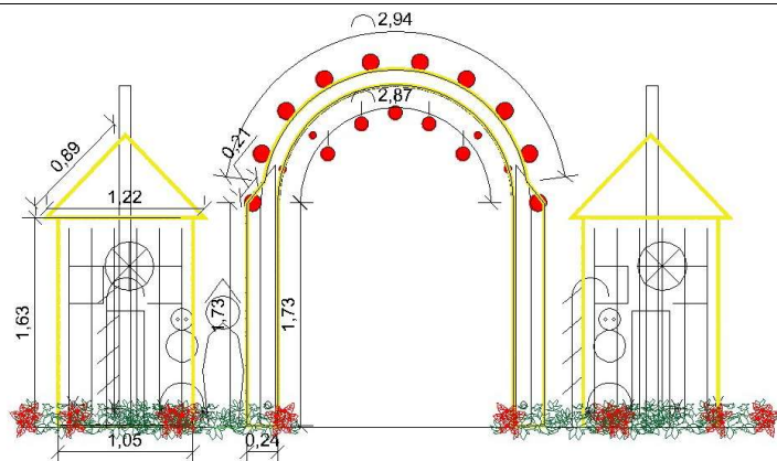
PORTAL NATAL - ELEVÇÃO ESQUEMÁTICA
