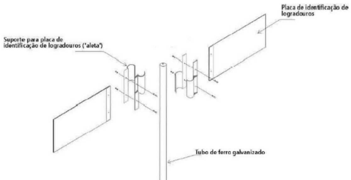
Figura 2 - Detalhe Fixação Placas de Identificação de Rua
