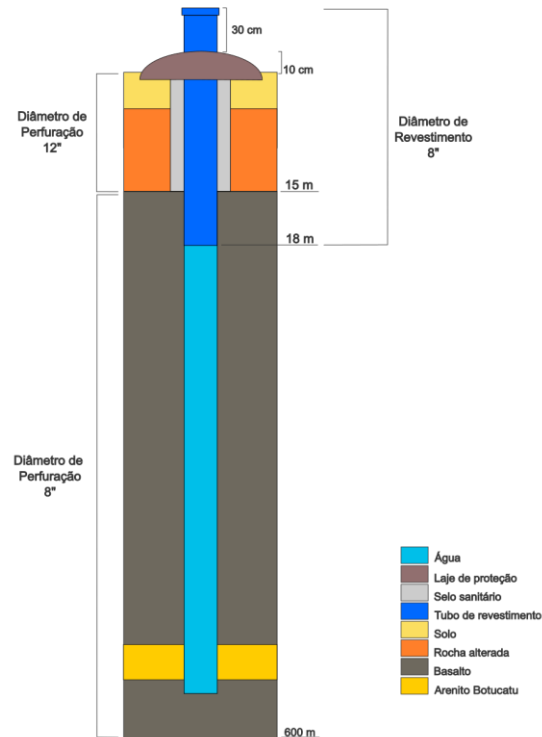
Figura 3: Perfil geológico e construtivo do poço
