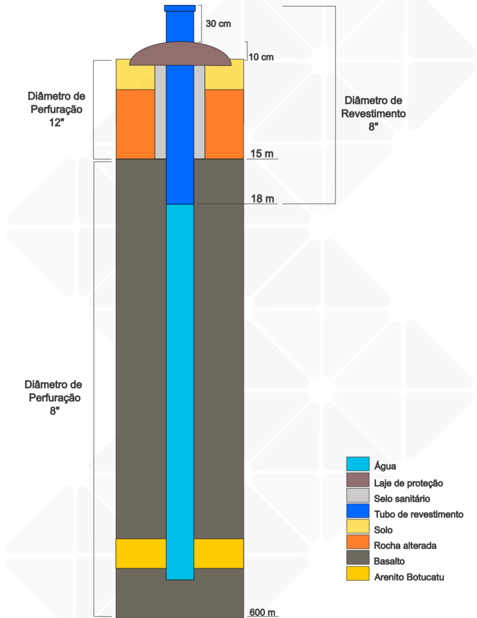
Figura 3: Perfil geológico e construtivo do poço
