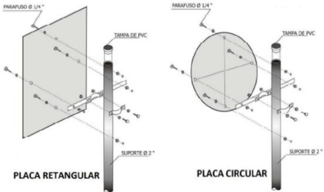
FONTE: Especificações Técnicas de Sinalização Vertical (BHTrans, 2013)
