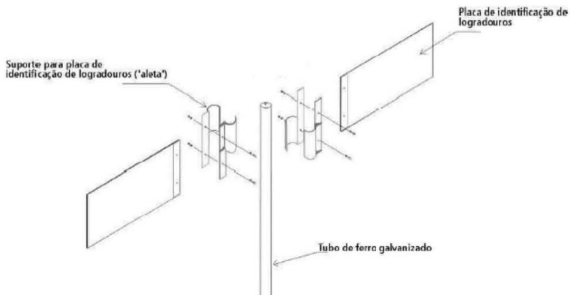
FONTE: Especificações de Concorrência Pública - EMURB (PMSP, 2005)
