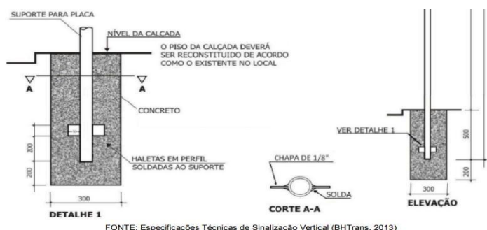
Figura 3 - Detalhe do Dispositivo Anti-Giro e da Fundação
