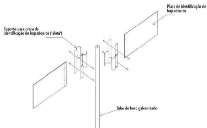
Figura 2 - Detalhe Fixação Placas de Identificação de Rua
