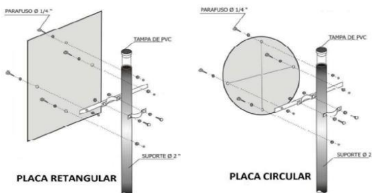
Figura 1 - Detalhe Fixação Placas
