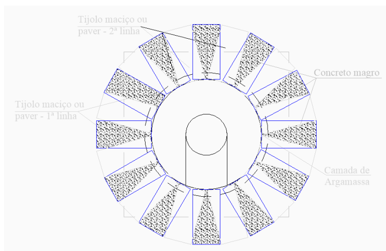
Vista em planta do assentamento dos tijolos/pavers
