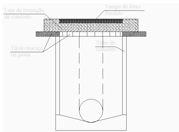
Vista em corte do assentamento dos tijolos/pavers
