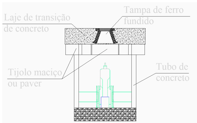
Vista em corte do assentamento dos tijolos/pavers
