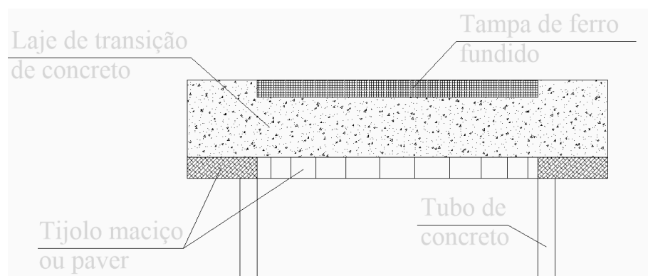
Vista em corte do assentamento dos tijolos/pavers
