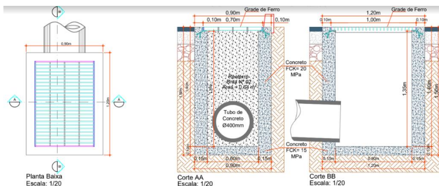
Imagem 01 – Detalhe Generico Bocas de lobo
