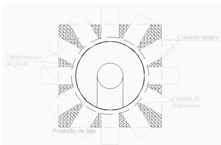
Vista em planta do assentamento dos tijolos/pavers
