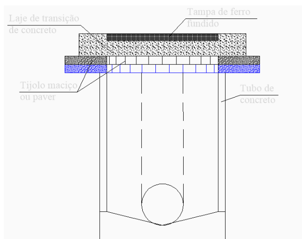
Vista em corte do assentamento dos tijolos/pavers
