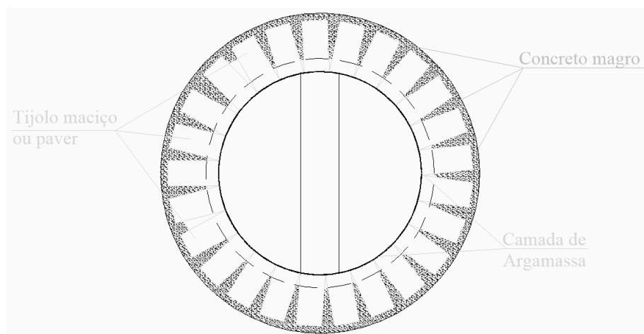
Vista em planta do assentamento dos tijolos/pavers
