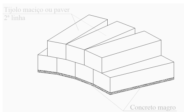
Posição dos tijolos/pavers
