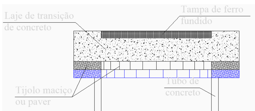
Vista em corte do assentamento dos tijolos/pavers
