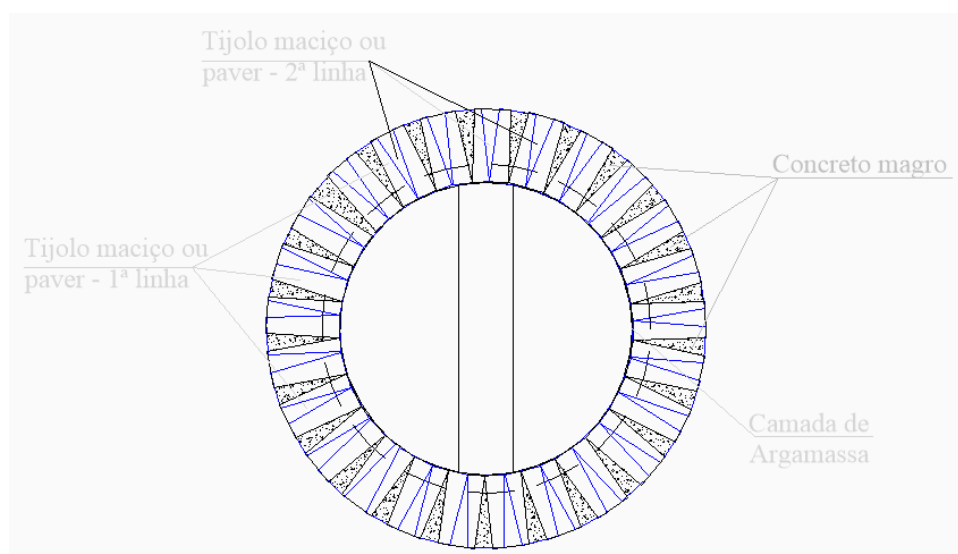
Vista em planta do assentamento dos tijolos/pavers
