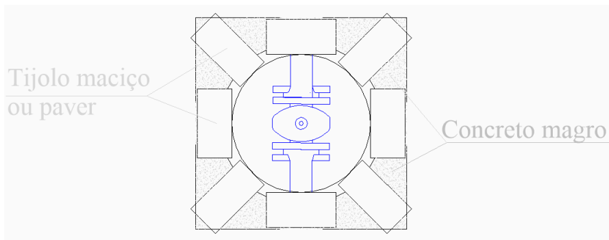
Vista em planta do assentamento dos tijolos/pavers
