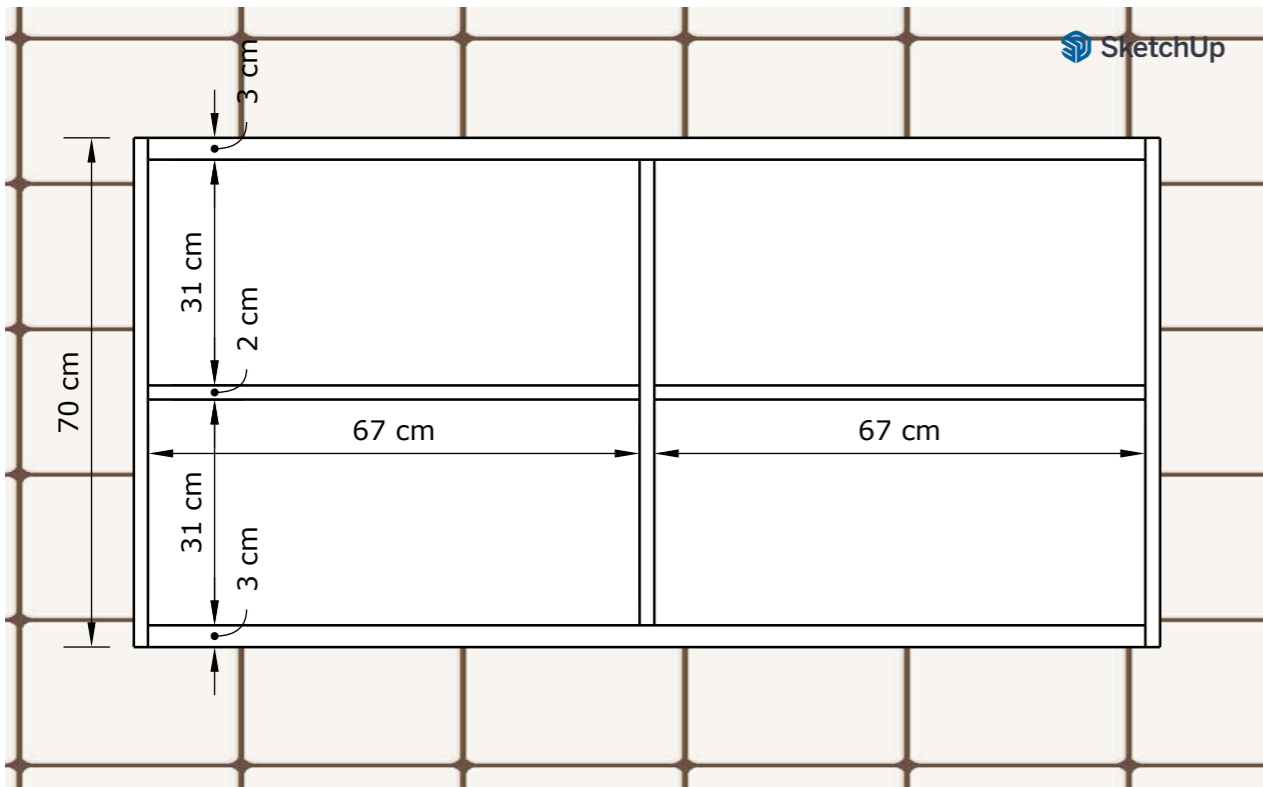
BALCÃO AÉREO - VISTA FRONTAL INTERNA
