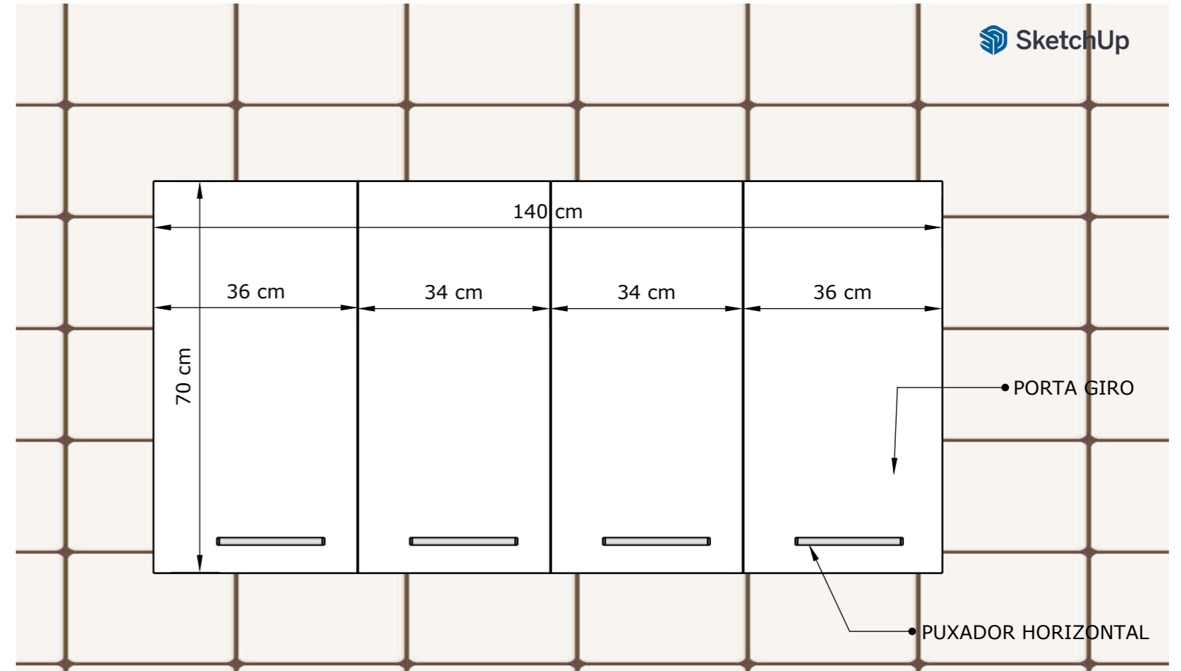
BALCÃO AÉREO - VISTA FRONTAL
