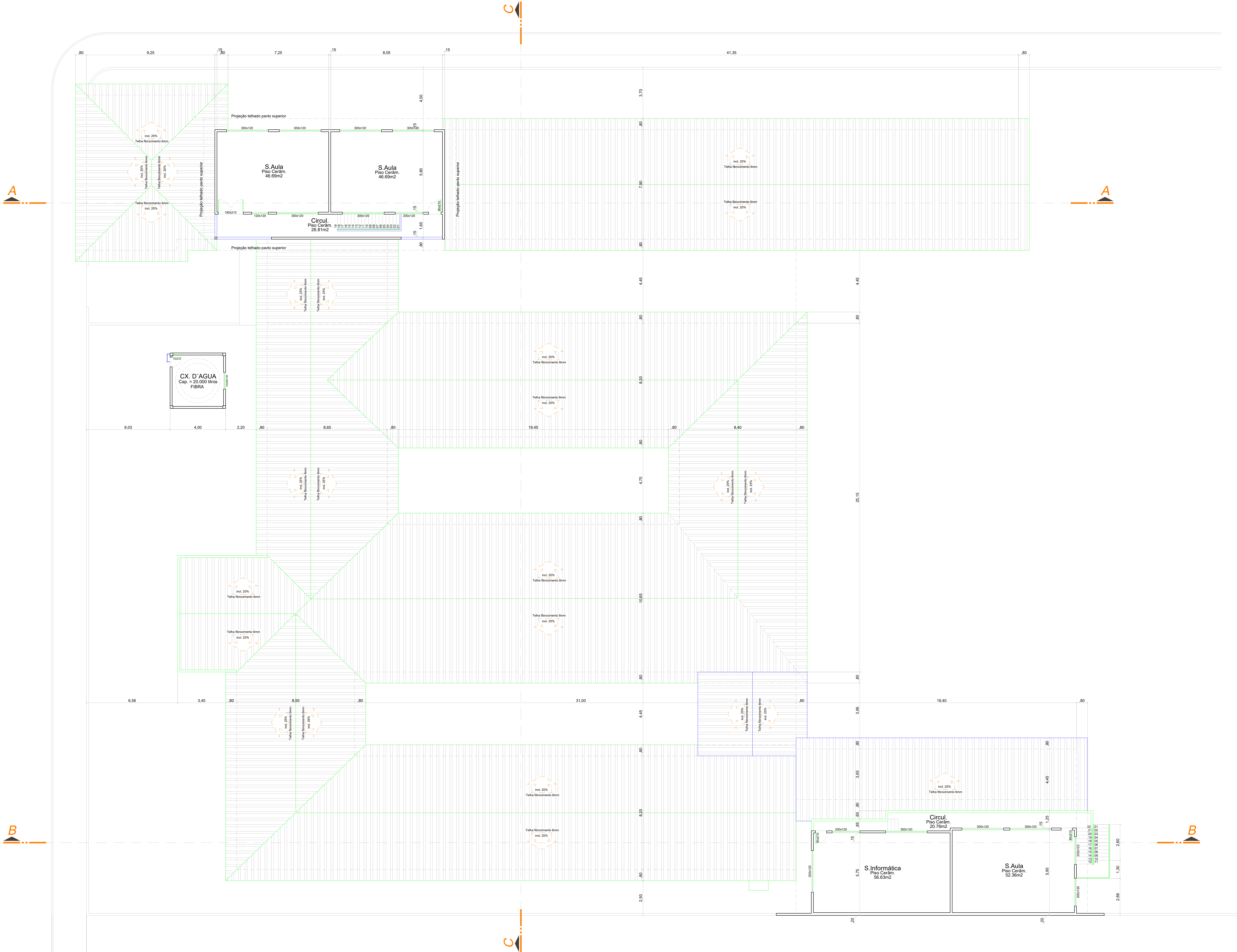
PL. BAIXA PAVTO SUPERIOR/TELHADO ESC. 1:100
