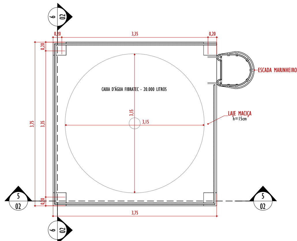
3 PLANTA BAIXA - PAVIMENTO LAJE 1 : 50
