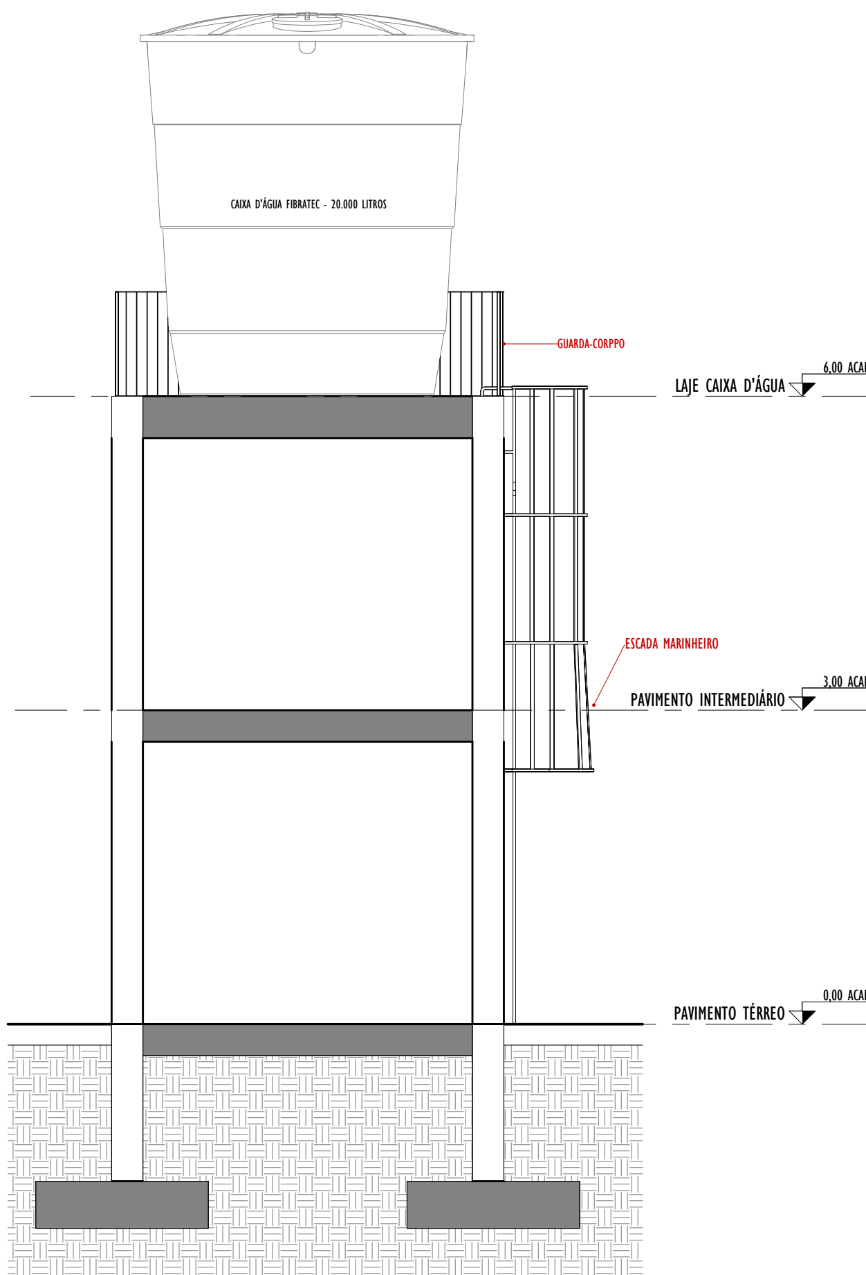
5 CORTE 5 1 : 50
