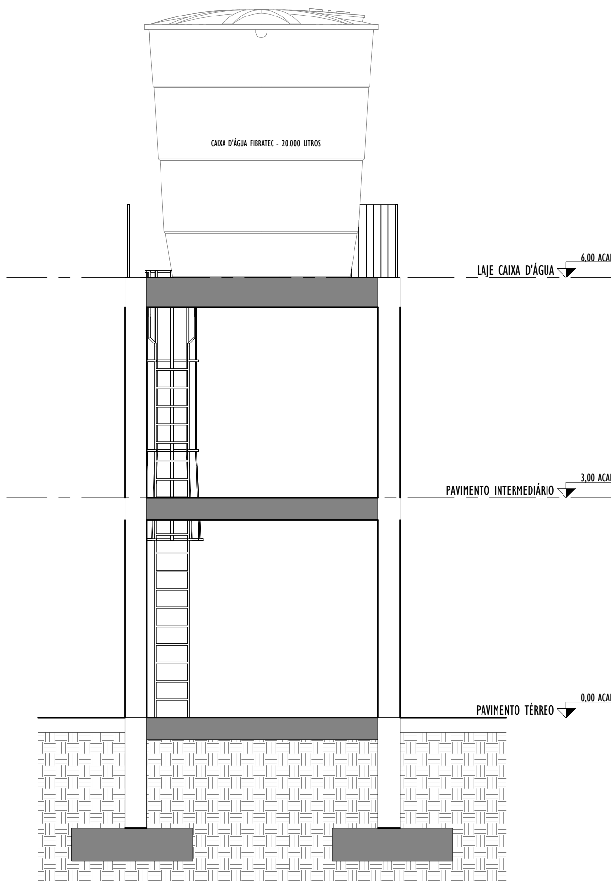
6 CORTE 6 1 : 50
