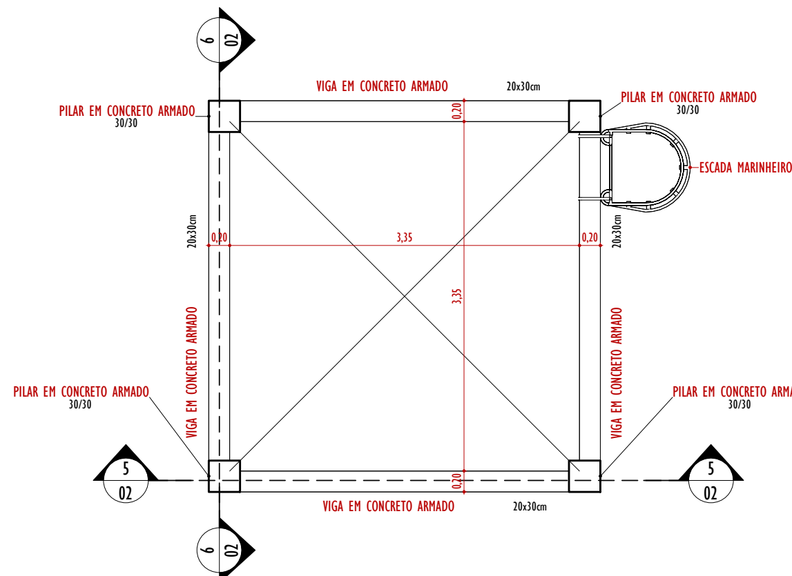
2 PLANTA BAIXA - PAV. INTERMEDIÁRIO 1 : 50
