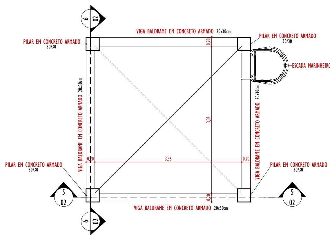
1 PLANTA BAIXA - PAV. TÉRREO 1 : 50
