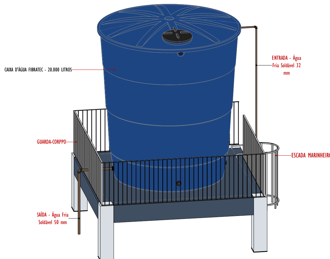
7 DETALHE CAIXA D'ÁGUA
