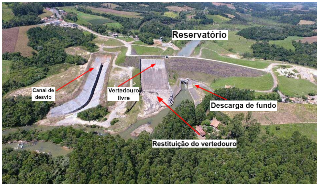
Figura 01 - Arranjo geral da barragem Sul
