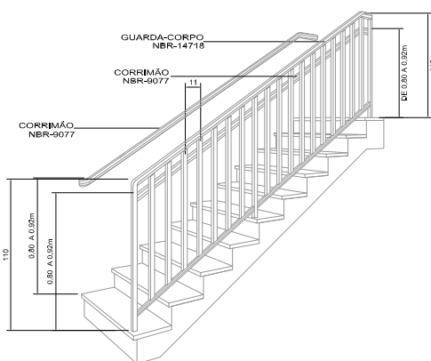
Detalhe Genérico Guarda Corpo e Corrimão Escadas e Rampas Esc.: 1/25
