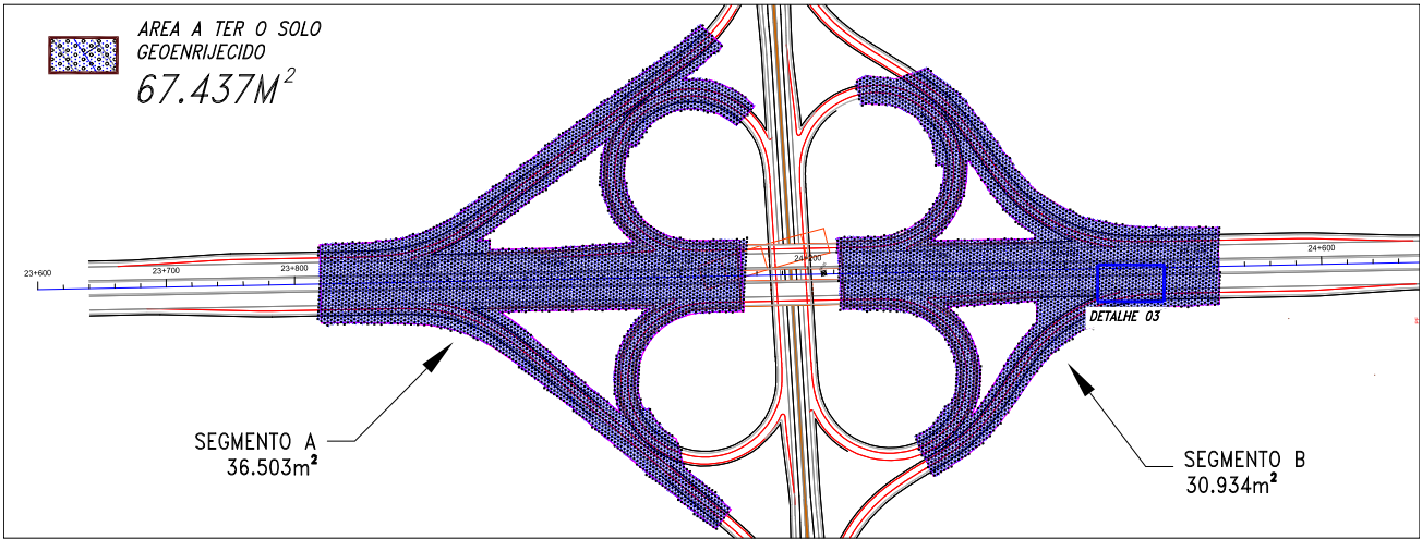
Figura 14 – Vista em Planta do Segmento P|04 - SC-486.
