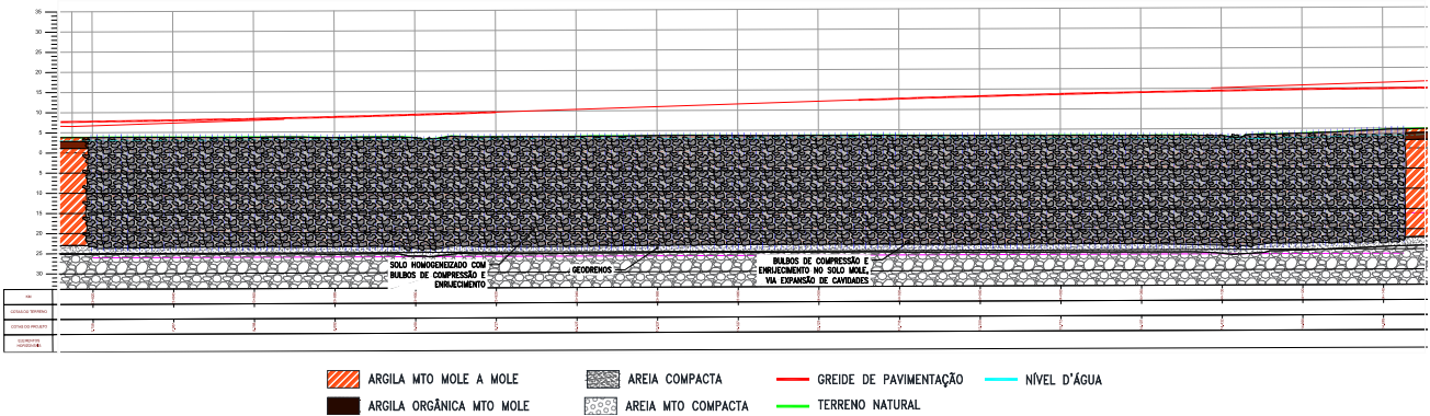
Figura 15 – Perfil geológico geotécnico do Segmento P|04 - SC-486, relativo a área de 36.503m².
