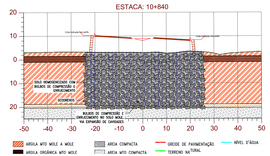
Figura 13 – Corte transversal da Estaca 10+840 com Geoenrijecimento.
