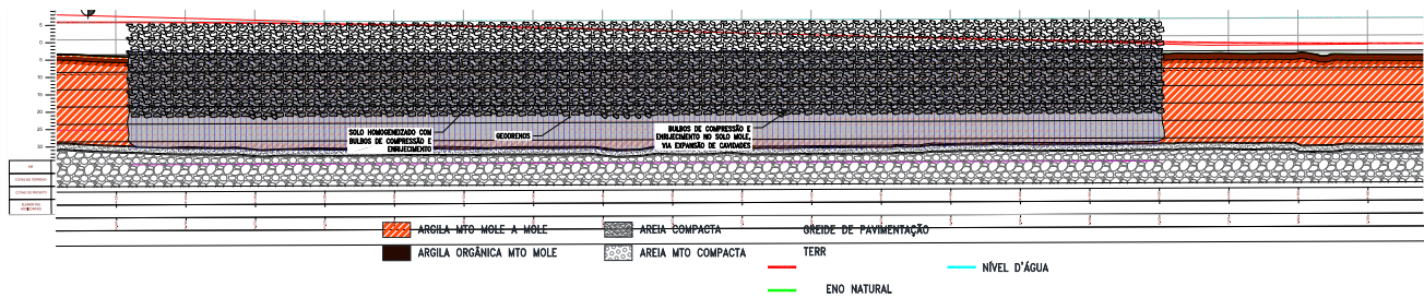
Figura 16 – Perfil geológico geotécnico do Segmento P|04 - SC-486, relativo a área de 30.934m².
