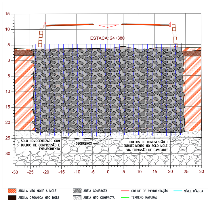
Figura 17 – Corte transversal da Estaca 24+380 com Geoenrijecimento.
