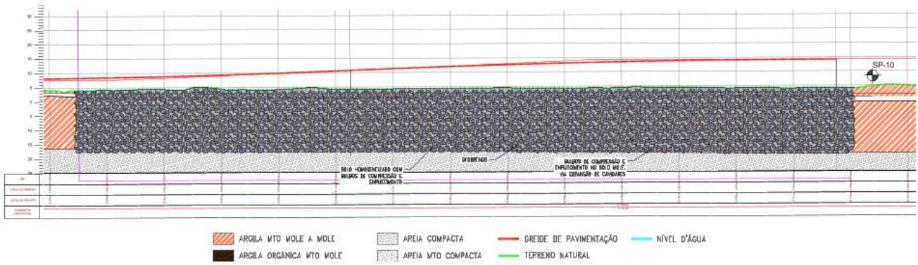
Figura 05 – Perfil geológico geotécnico do Segmento P|02 - BR-470 com Geoenriecimento, relativo a área de 17.700m 2 .
