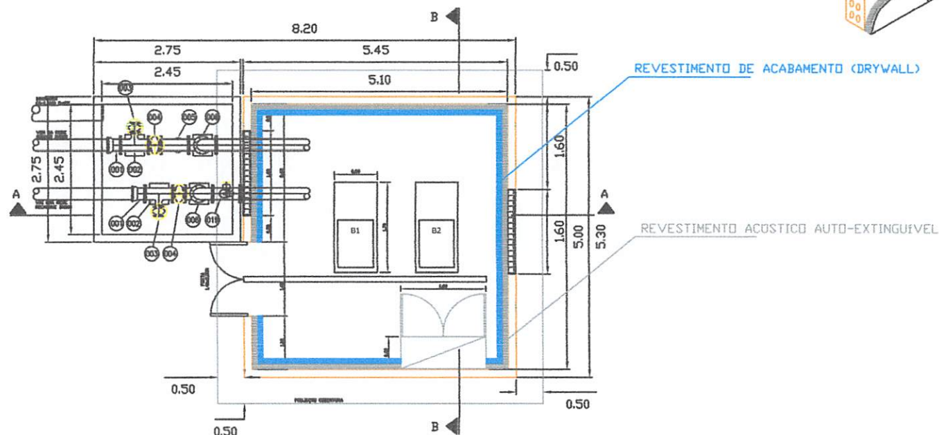
PLANTA BAIXA
