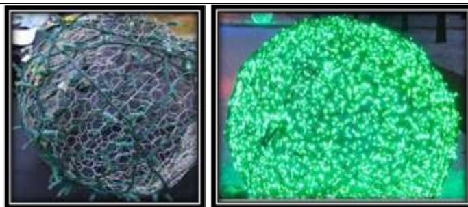
Figura 16 – Modelo da estrutura em formato de bola contornada por cordão luminoso de led, e a segunda imagem demonstra efeito luminoso desejado
