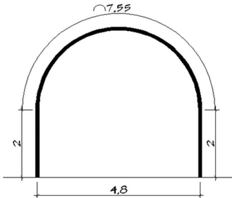
Figura 26 – Formato da estrutura metálica
