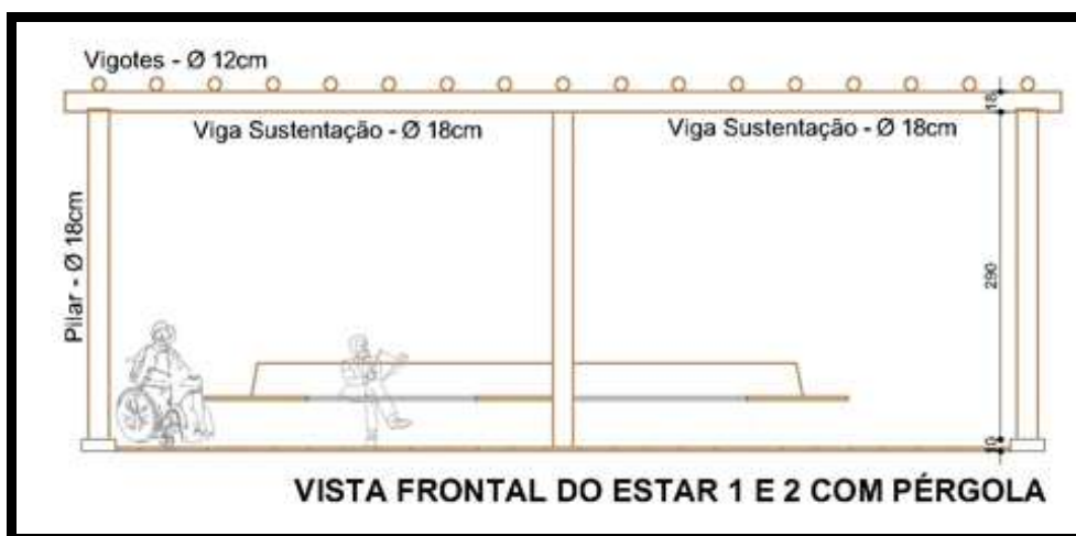
Figura 12 – Vista Frontal do Estar 1 e 2 com Pérgola, demonstrando a locação das Vigas de Sustentação, Vigotes apoiados sob as Vigas e Pilares
