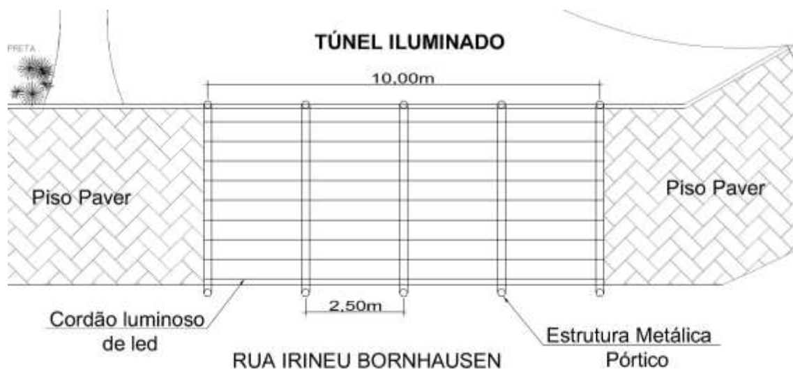
Figura 25 – Planta Baixa do posicionamento da estrutura metálica do Túnel e locação do mesmo sob o piso de paver
