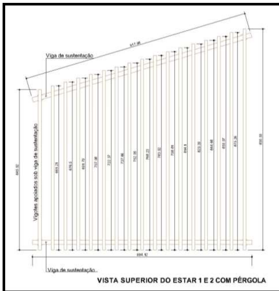
Figura 11 – Vista Superior do Estar 1 e 2 com Pérgola, demonstrando a locação das Vigas de Sustentação e Vigotes apoiados sob as Vigas
