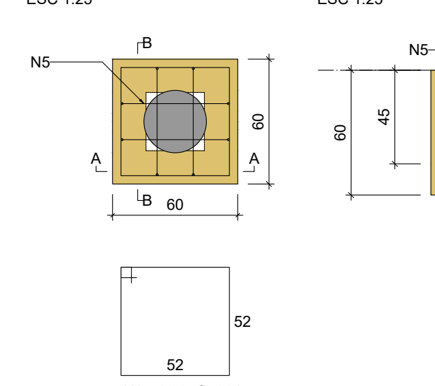
B30 1xC30 PLANTA ESC 1:25
