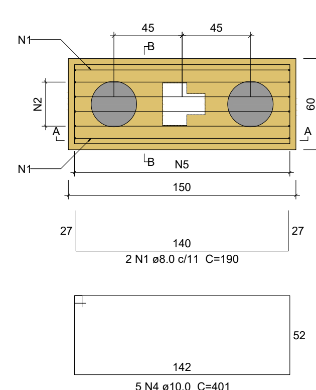
B15 2xC30 PLANTA ESC 1:25
