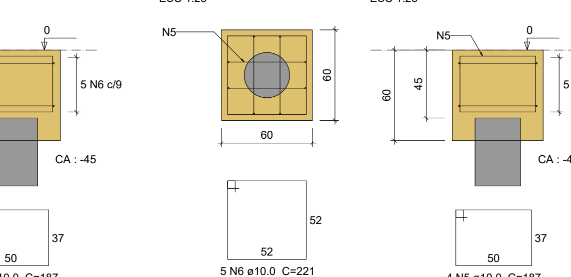
B18 1xC30 PLANTA ESC 1:25
