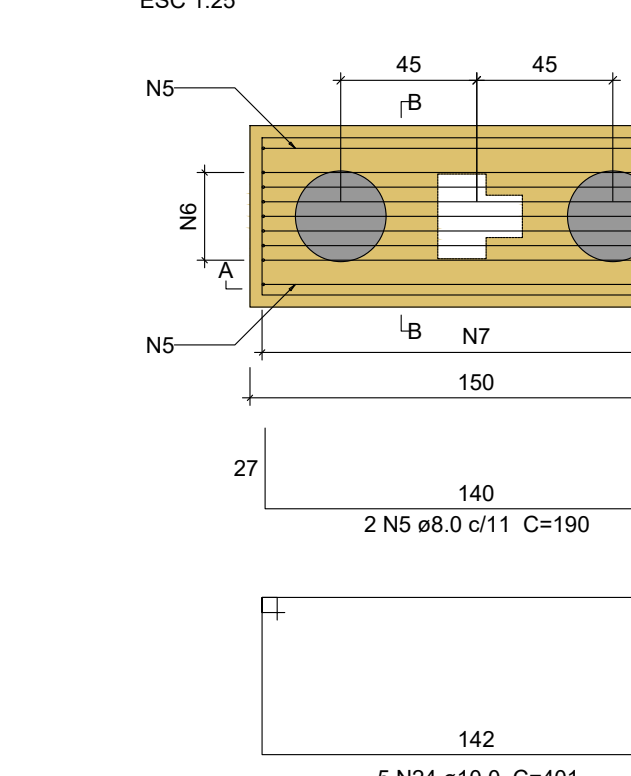
B33 2xC30 PLANTA ESC 1:25
