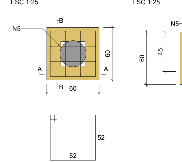
B31 1xC30 PLANTA ESC 1:25
