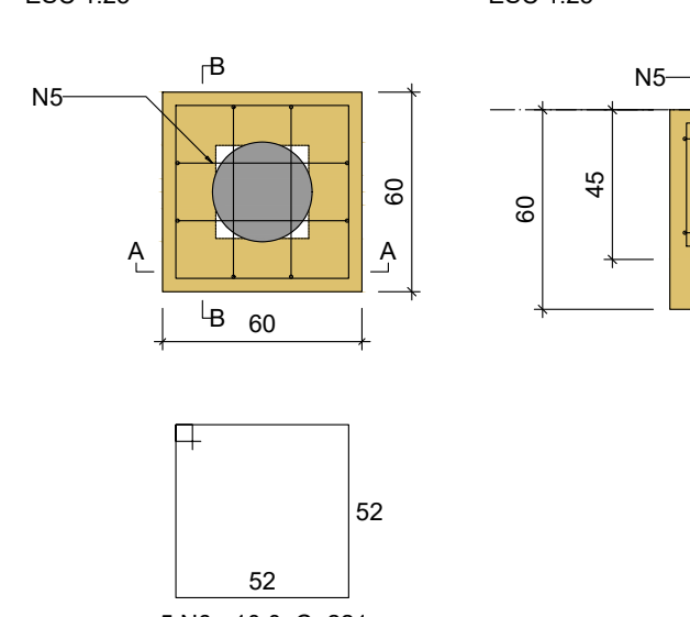
B27 1xC30 PLANTA ESC 1:25
