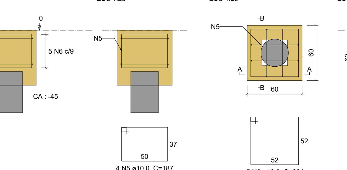
B27 1xC30 PLANTA ESC 1:25
