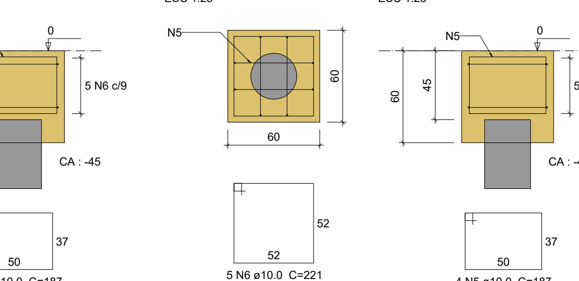
B19 1xC30 PLANTA ESC 1:25
