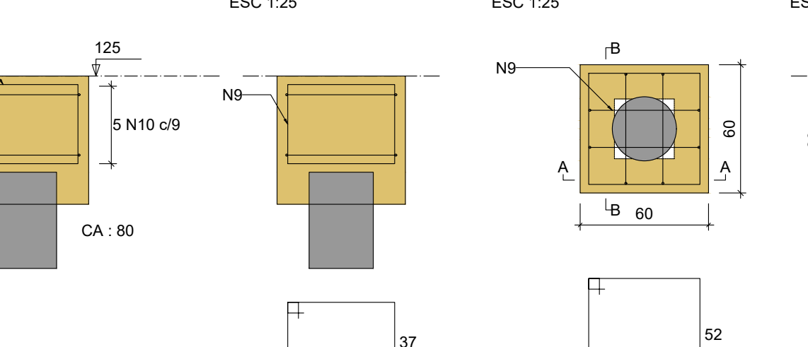
B36 1xC30 PLANTA ESC 1:25
