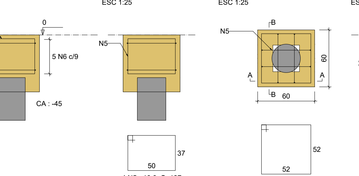
B30 1xC30 PLANTA ESC 1:25
