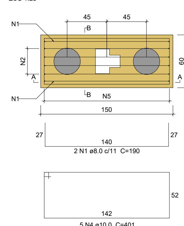
B21 1xC30 PLANTA ESC 1:25
