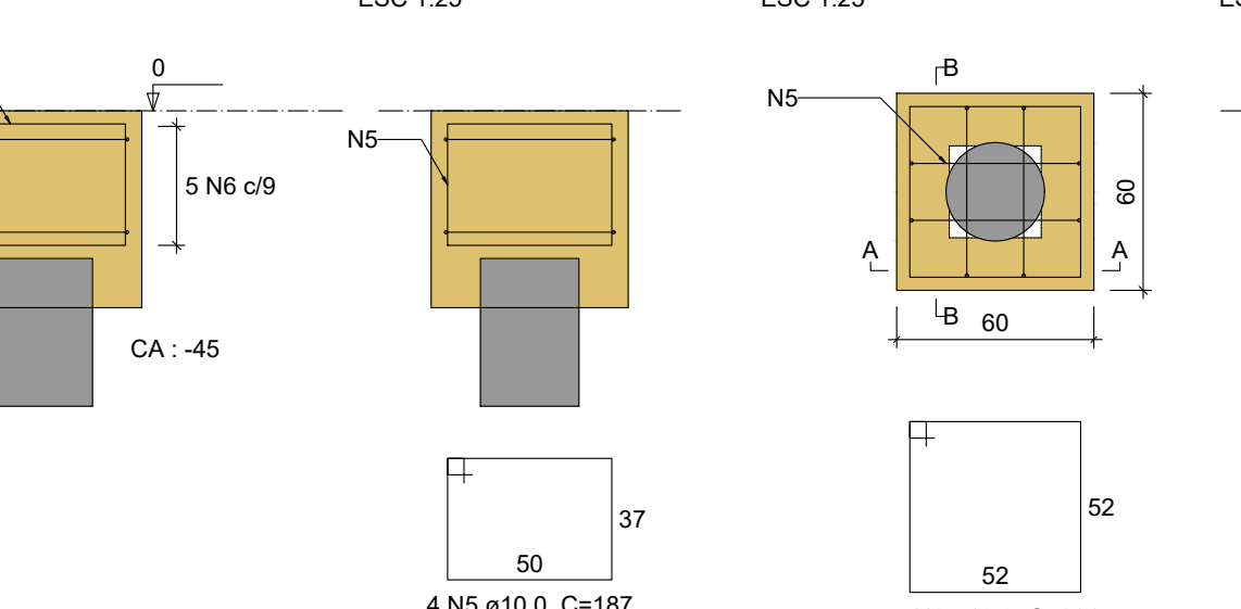
B31 1xC30 PLANTA ESC 1:25
