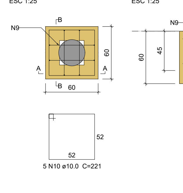
B36 1xC30 PLANTA ESC 1:25
