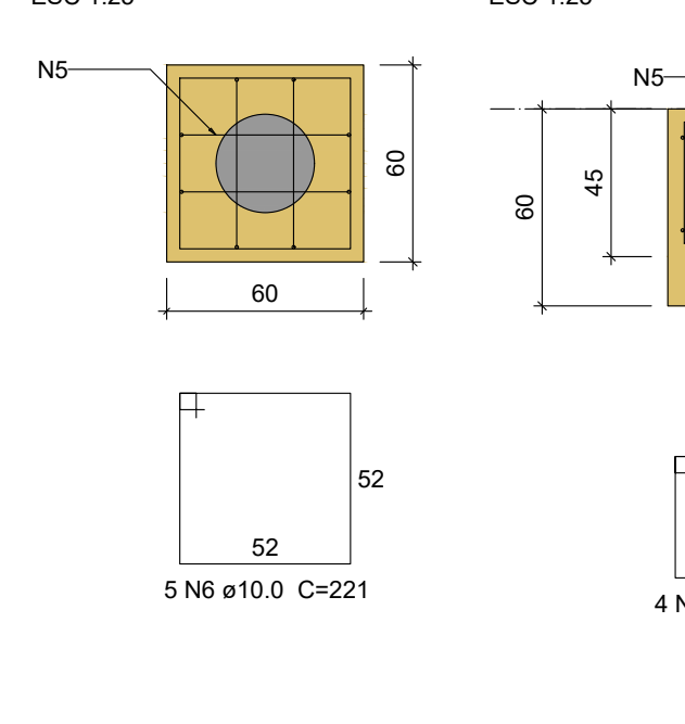
B23 1xC30 PLANTA ESC 1:25
