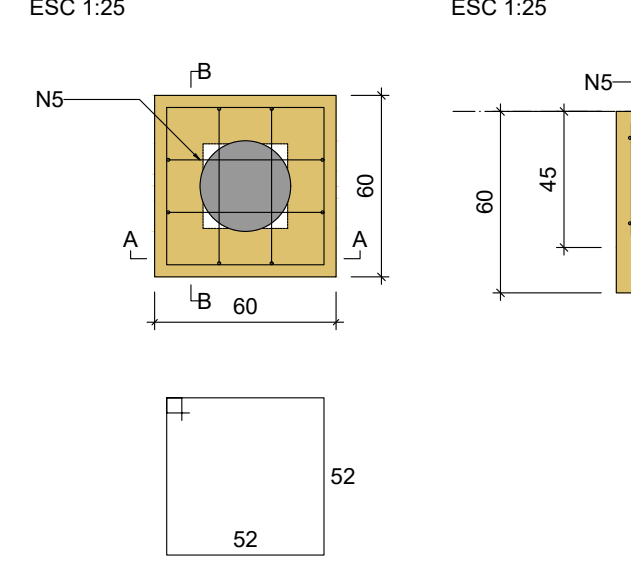
B29 1xC30 PLANTA ESC 1:25
