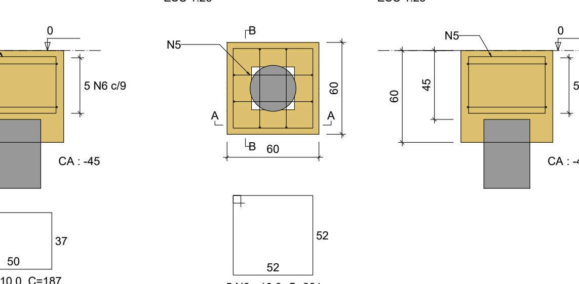
B26 1xC30 PLANTA ESC 1:25
