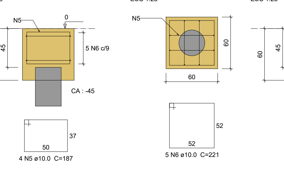
B24 1xC30 PLANTA ESC 1:25
