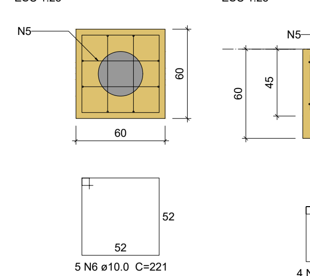
B25 1xC30 PLANTA ESC 1:25
