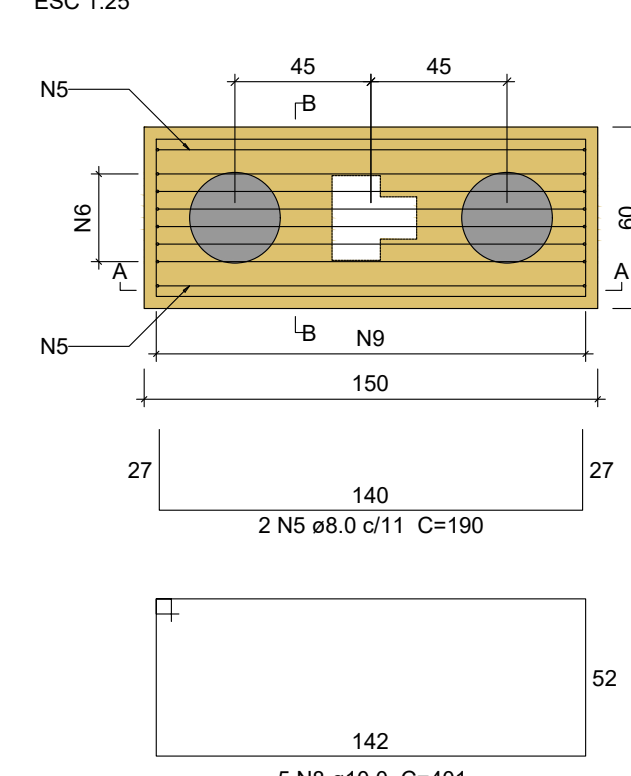
B34 2xC30 PLANTA ESC 1:25
