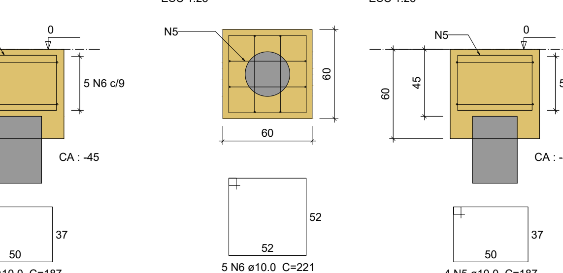
B20 1xC30 PLANTA ESC 1:25
