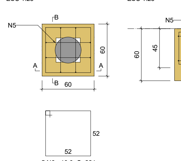
B28 1xC30 PLANTA ESC 1:25
