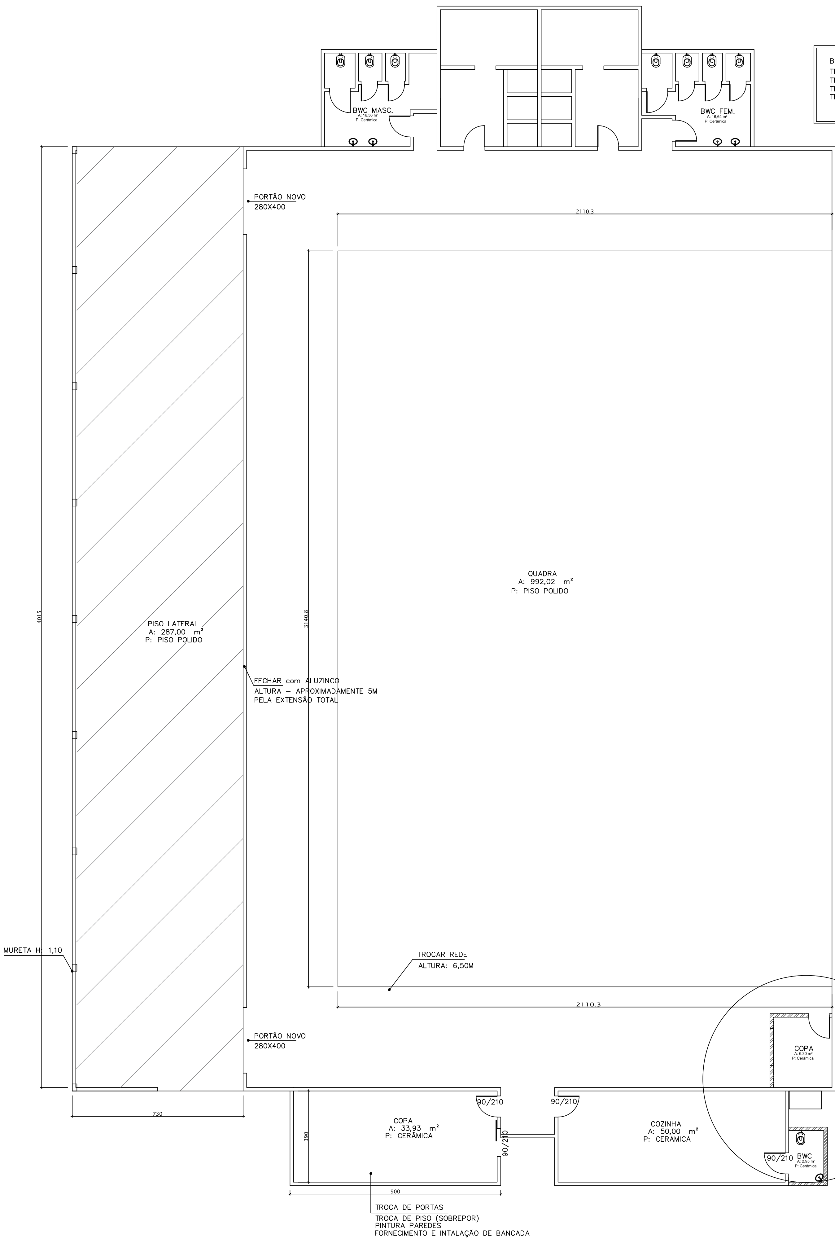
PLANTA BAIXA ESC.: 1/100
