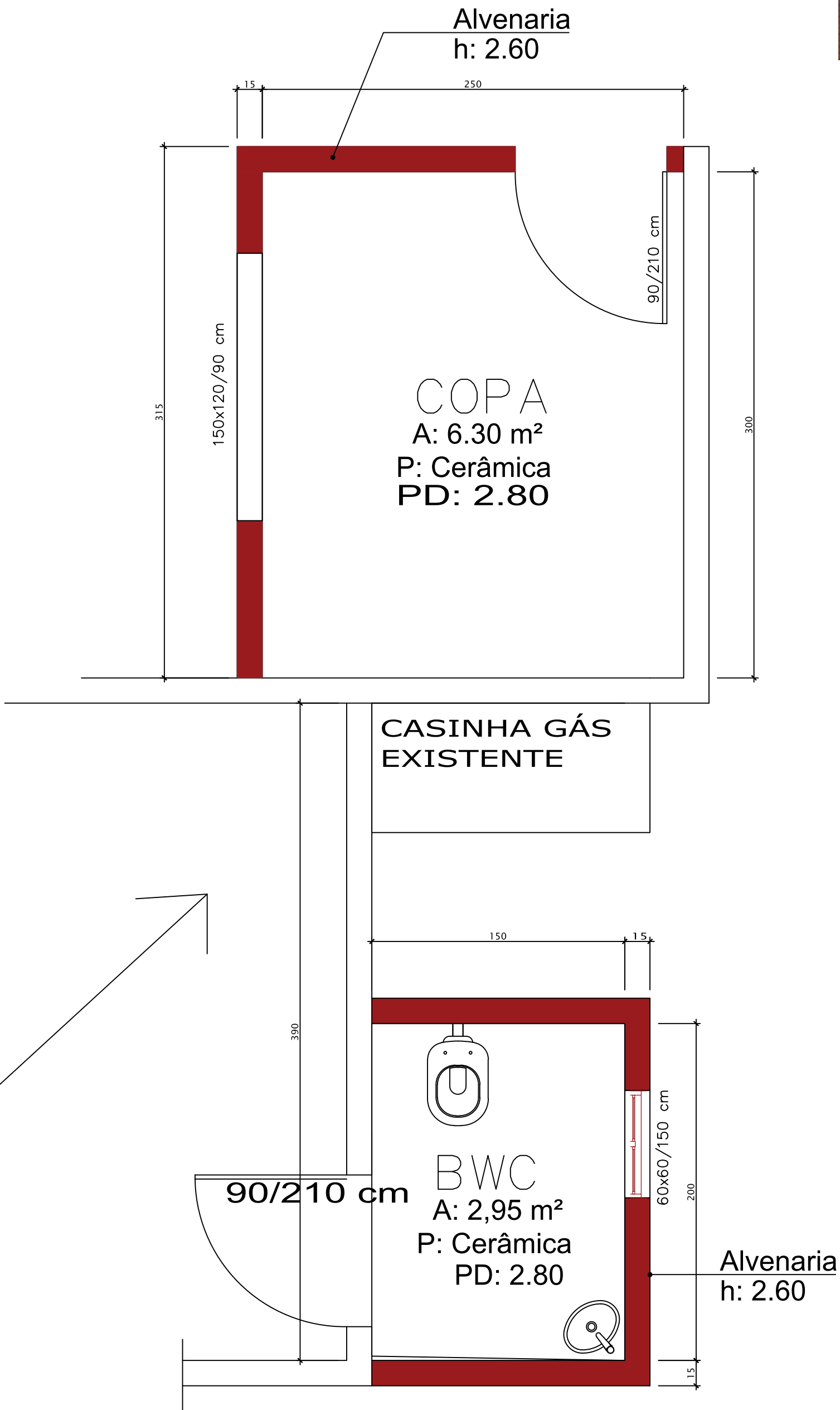
DETALHE COPA E BANHEIRO ESC.: 1/25
