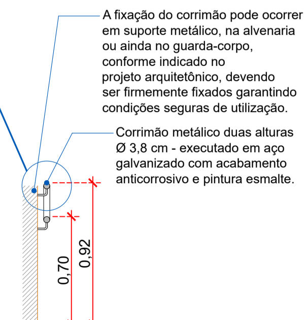
DETALHE CORRIMÃO Esc. 1/25
