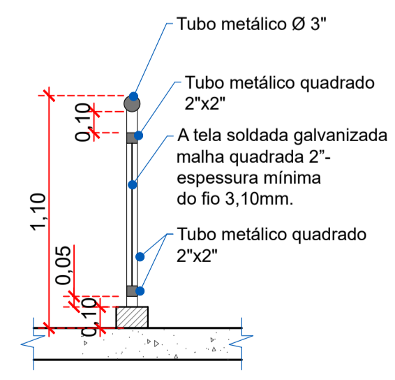
DETALHE GUARDA-CORPO PISTA BOLICHE E RAMPA INTERNA Esc. 1/25
