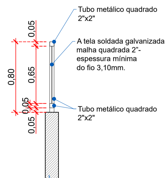
DETALHE PROTEÇÃO METÁLICA CANCHAS DE BOCHA Esc. 1/25
