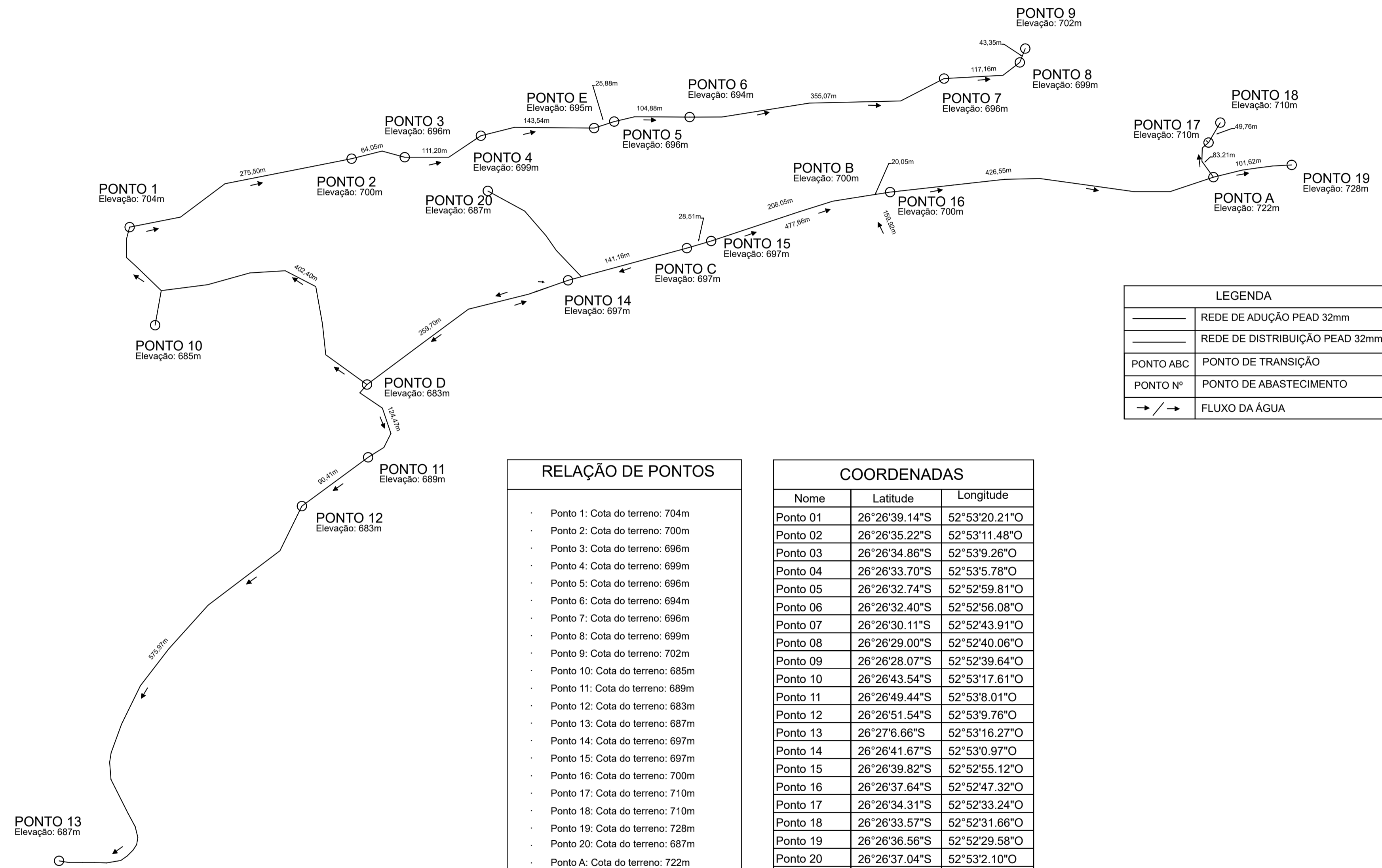
PLANTA BAIXA DE PONTOS SEM ESCALA
