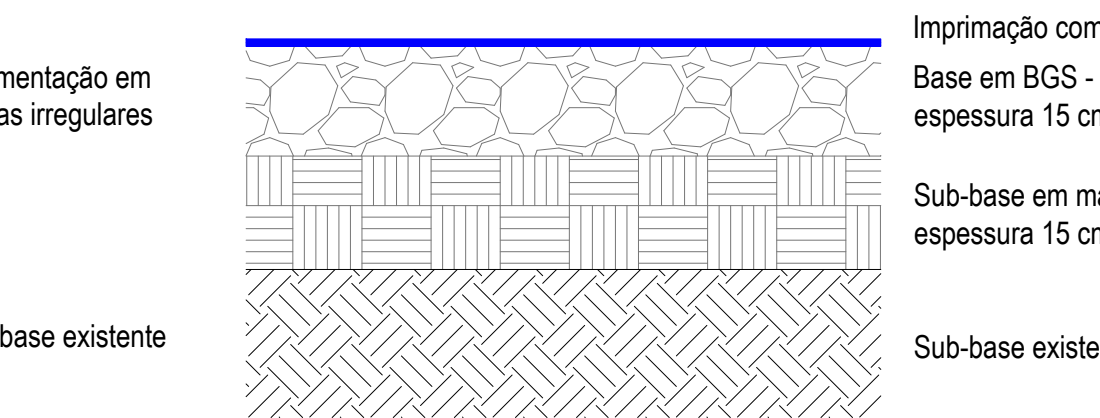
SEÇÃO DA VIA APÓS REFORÇO DO SUBLEITO
