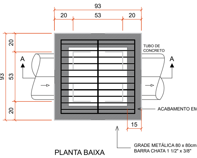
DETALHE 02 - CAIXA COLETORA C/BOCA DE LOBO - TUBO Ø40cm Escala 1:25
