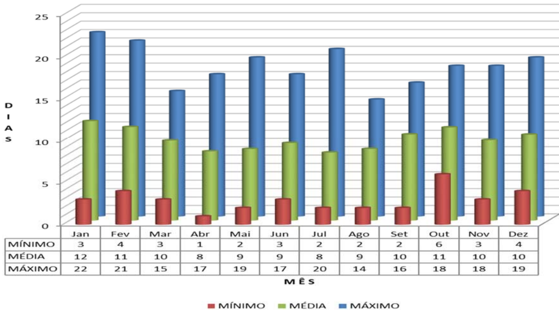
Figura 3-5 – Gráfico dos dias de Chuva
