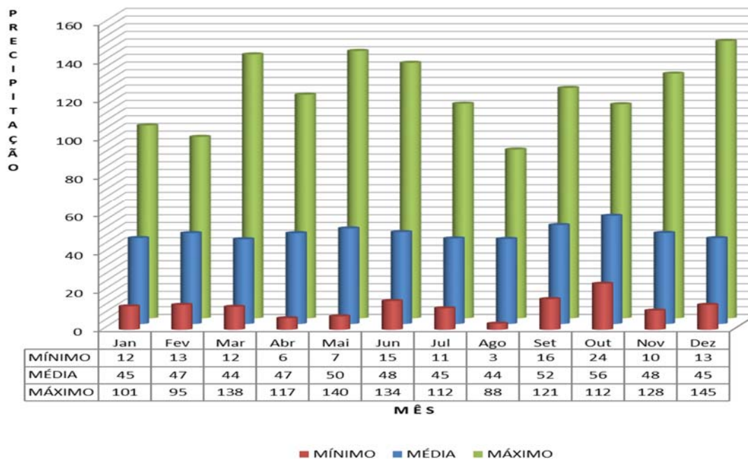
Figura 3-4 – Gráfico da Precipitação máxima mensal
