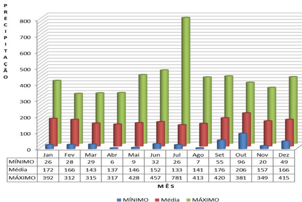
Figura 3-3 – Gráfico da Precipitação Total Mensal
