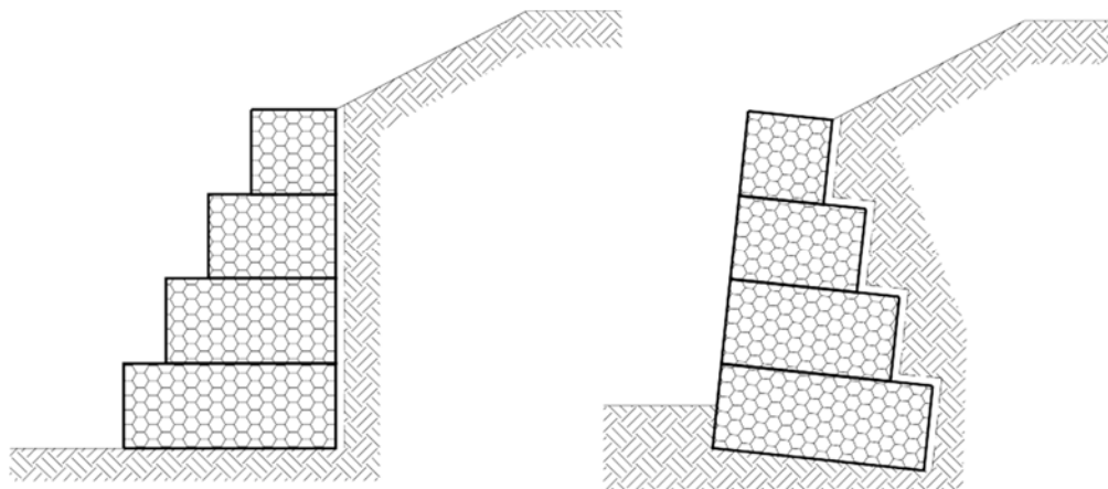
Figura 4-1- Muro de gabiões com degraus externos e com degraus internos
