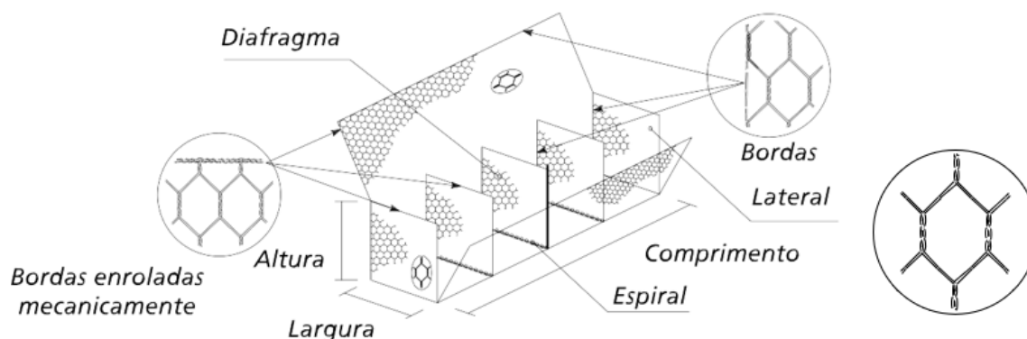
Figura 4-2- Elementos constituintes dos gabiões tipo caixa
