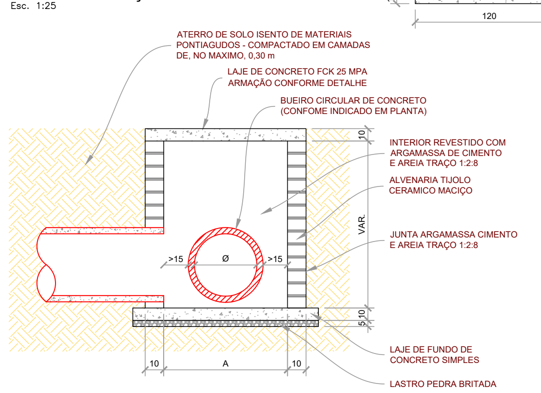
CAIXA DE LIGAÇÃO - CORTE AA
