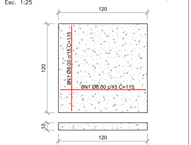
LAJE SUPERIOR CAIXA DE LIGAÇÃO
