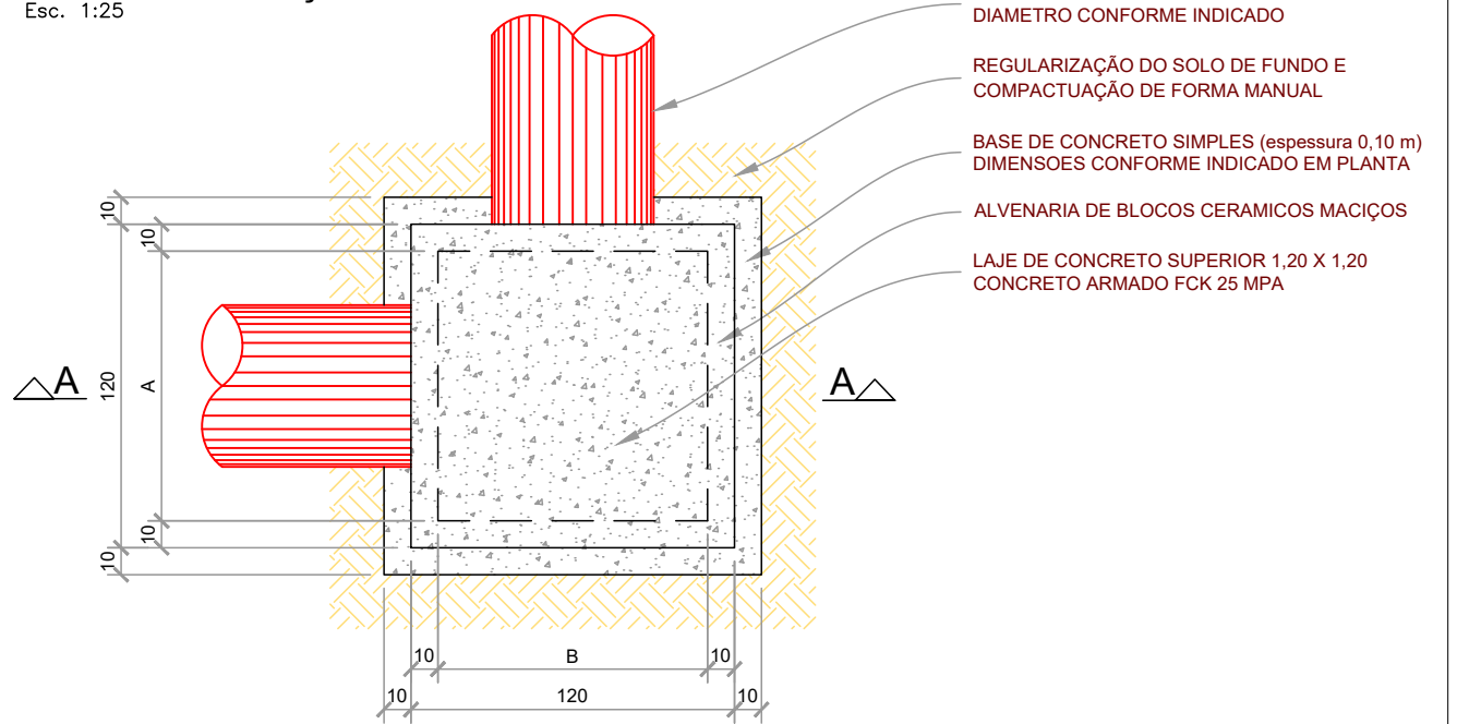
LAJE SUPERIOR CAIXA DE LIGAÇÃO
