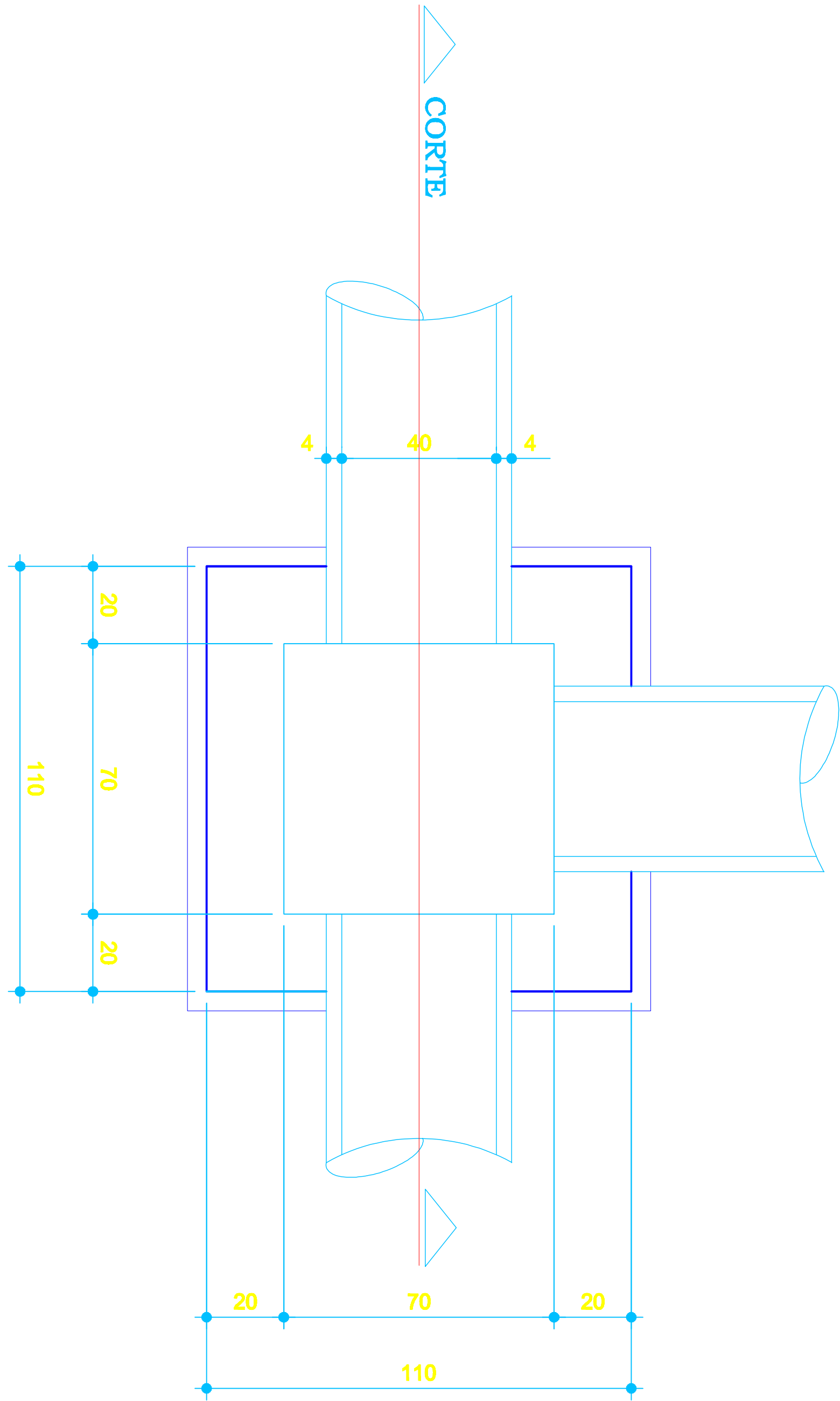
Planta Baixa Caixa de Ligação Tubo Ø 40 Escala 1:25
