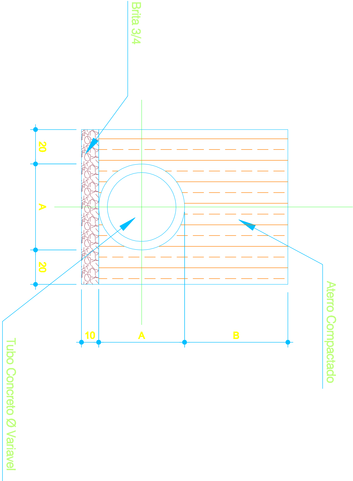
Assentamento de Tubulação Escala 1:25
