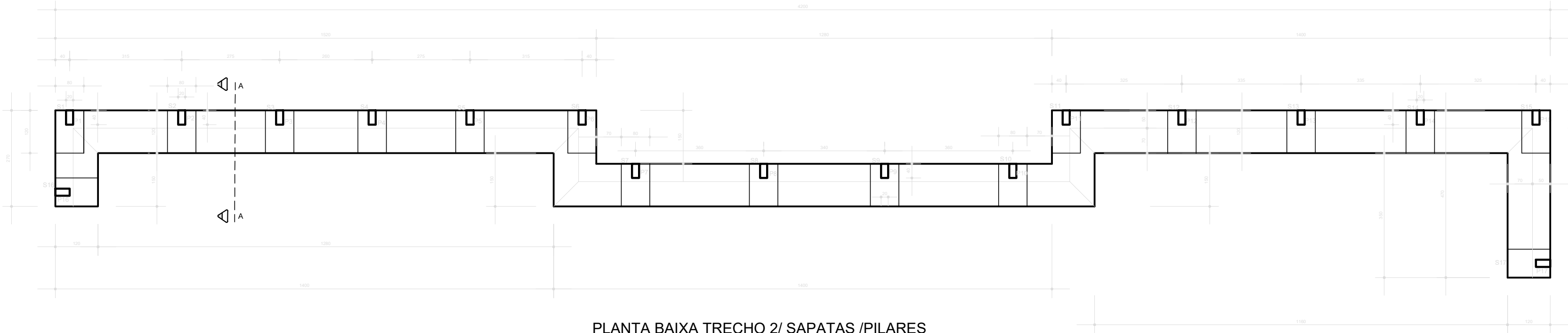
PLANTA BAIXA TRECHO 2/ SAPATAS /PILARES esc. 1:50
