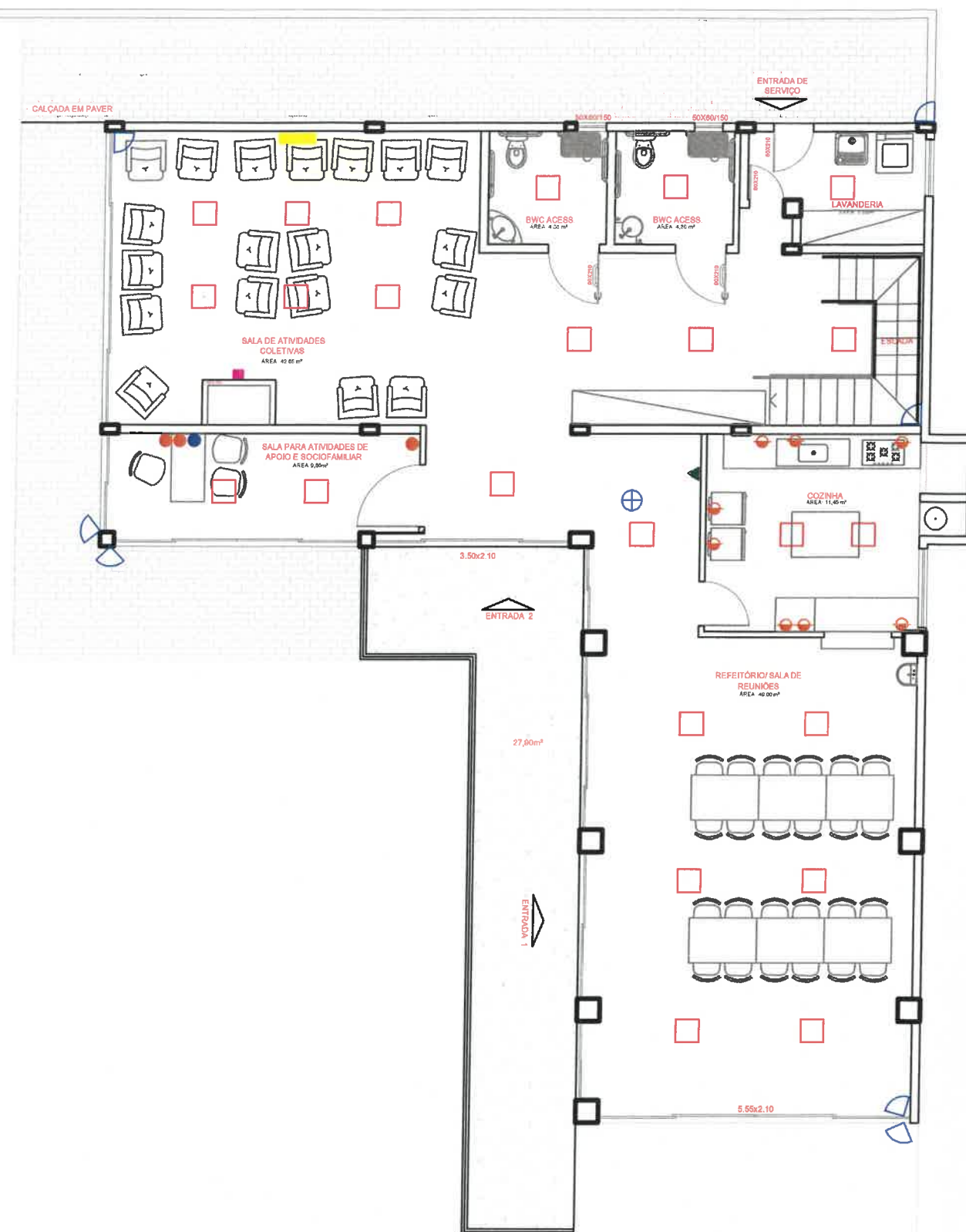
PLANTA BAIXA - PAV. INFERIOR, PONTOS DE ELÉTRICA E LÓGICA ESCALA 1:50
