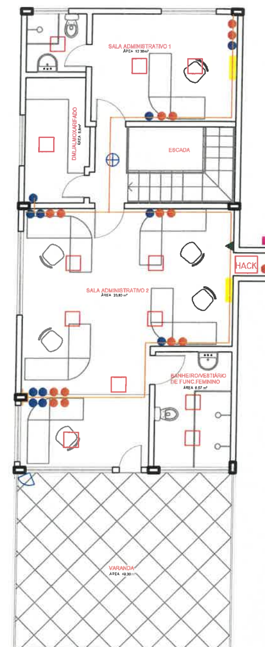
PLANTA BAIXA - PAV. SUPERIOR PONTOS DE ELÉTRICA E LÓGICA ESCALA 1:50
