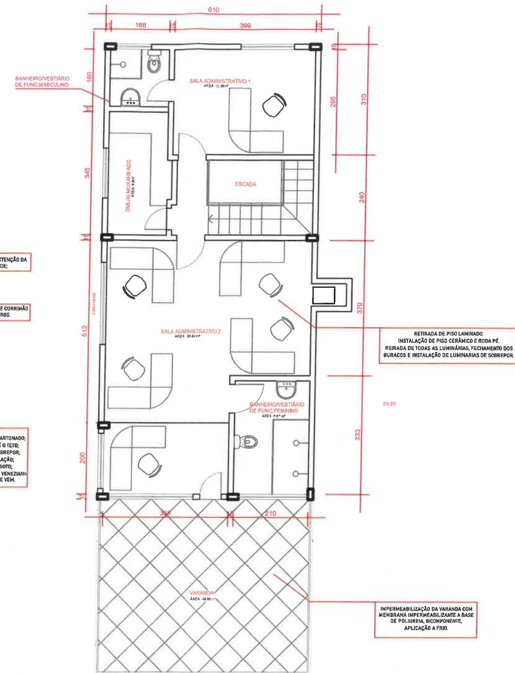
PLANTA BAIXA - PAV. SUPERIOR ESCALA 1:50
