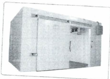
Câmara frigorífica com medidas e temperaturas de acordo com as necessidades do cliente, isolamento em PUR e EPS, acabamento em aço inox 304 e chapa aço pintura epóxi branca.
