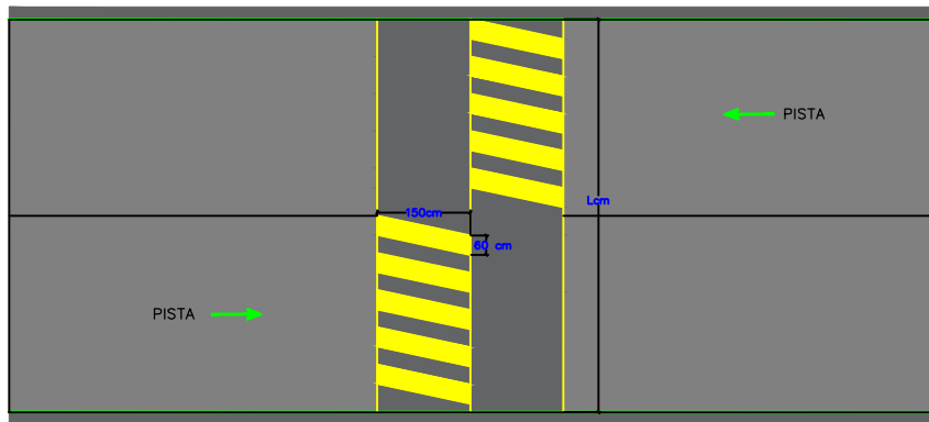
Detalhamento Lombada
