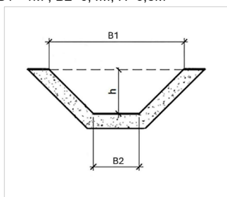
Detalhe da Canaleta
