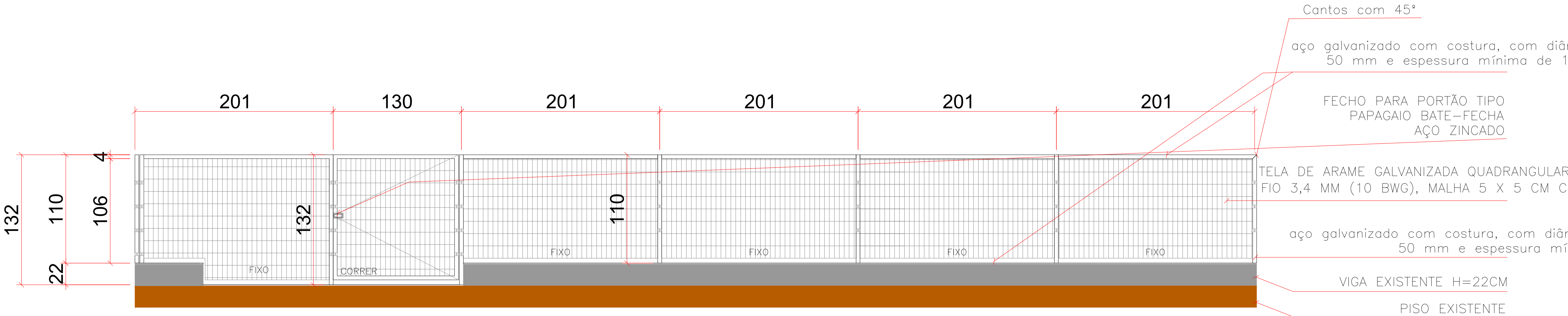
Elevação 1 - Gradil
