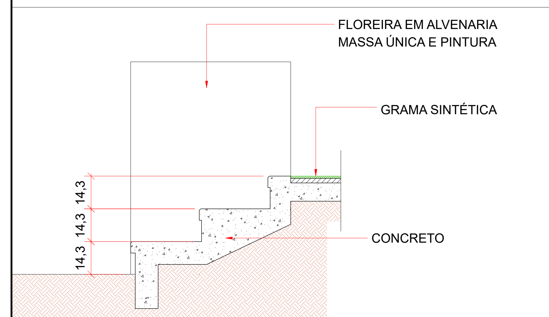
DETALHE ESCADA CONCRETO
