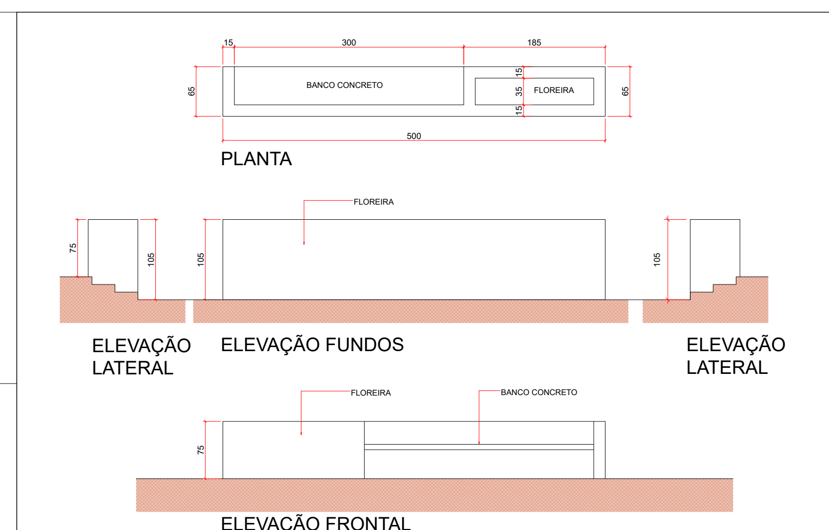
DETALHE BANCO ALVENARIA
