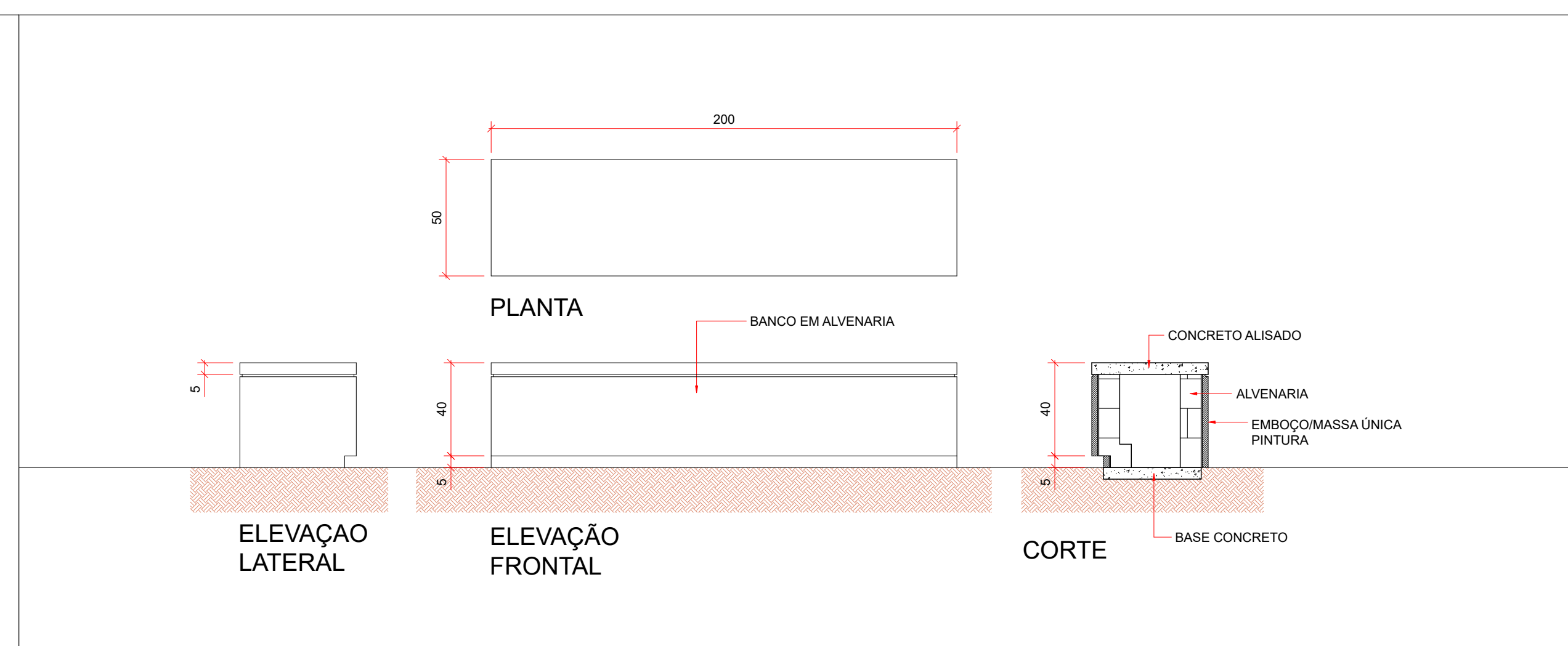
DETALHE BANCO ALVENARIA
