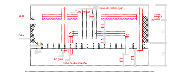
Filtro areia - PLOTTIS Cota 1 - ESC. 1,25
