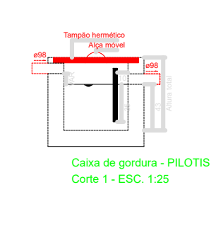
Caixa de gordura - PLOTTIS Planta baixa - ESC. 1,25
