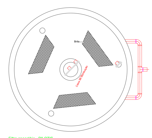
Filtro areia - PLOTTIS Planta baixa - ESC. 1,25
