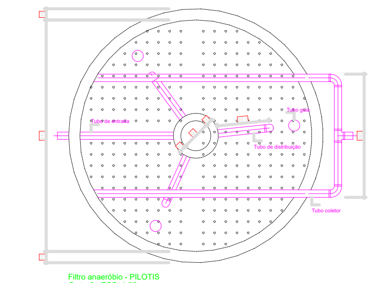
Filtro areia - PLOTTIS Cota 2 - ESC. 1,25
