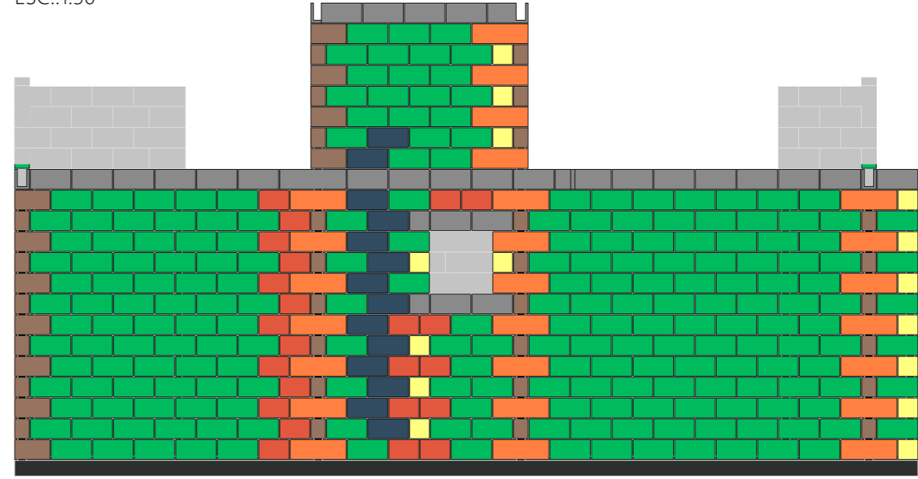
FACHADA 4 ESC.:1:50
