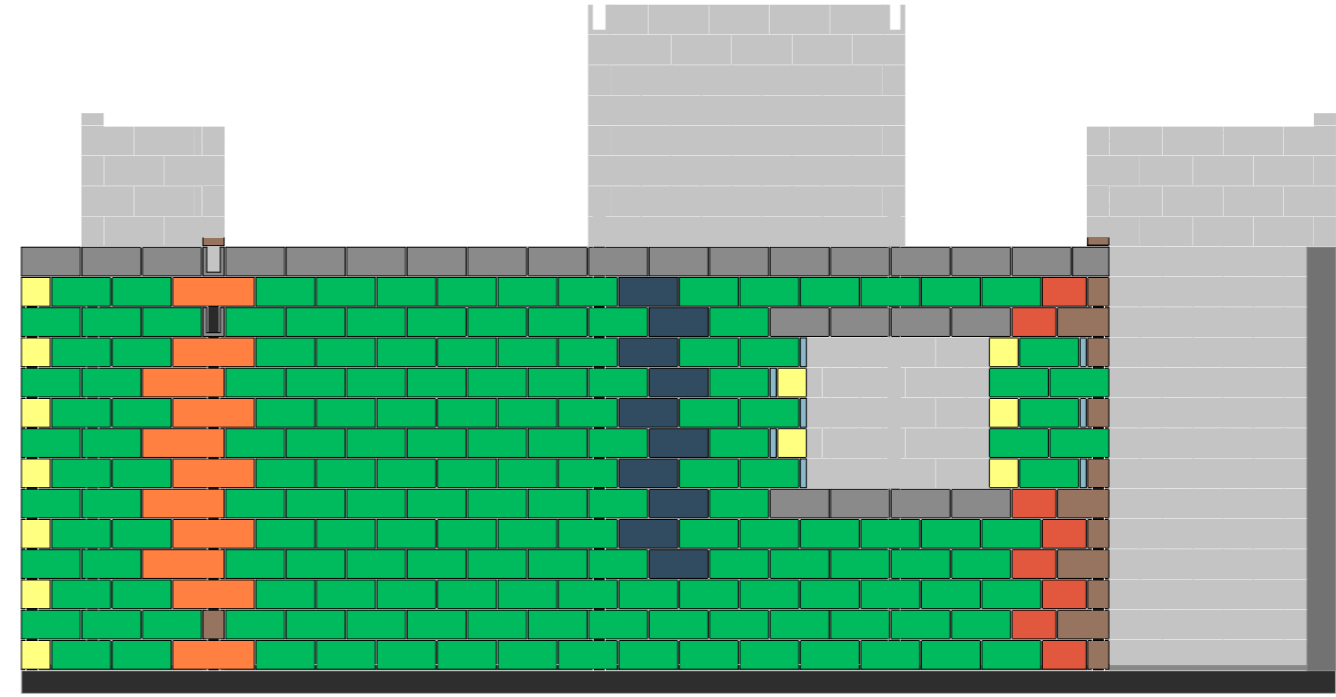
FACHADA 2 ESC.:1:50
