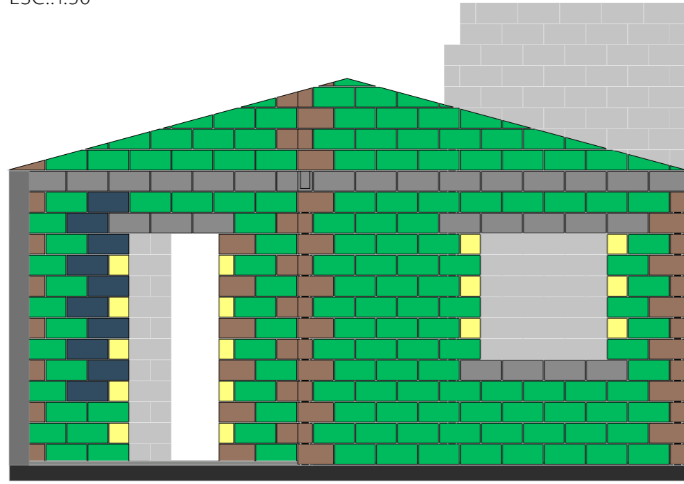
FACHADA 3 ESC.:1:50
