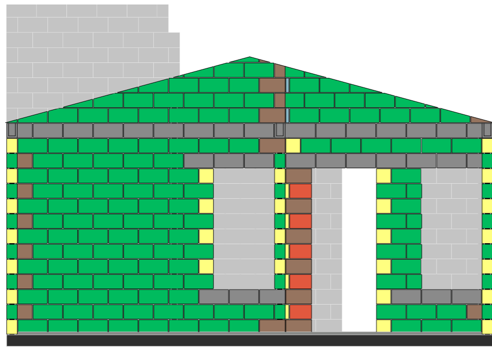
FACHADA 1 ESC.:1:50
