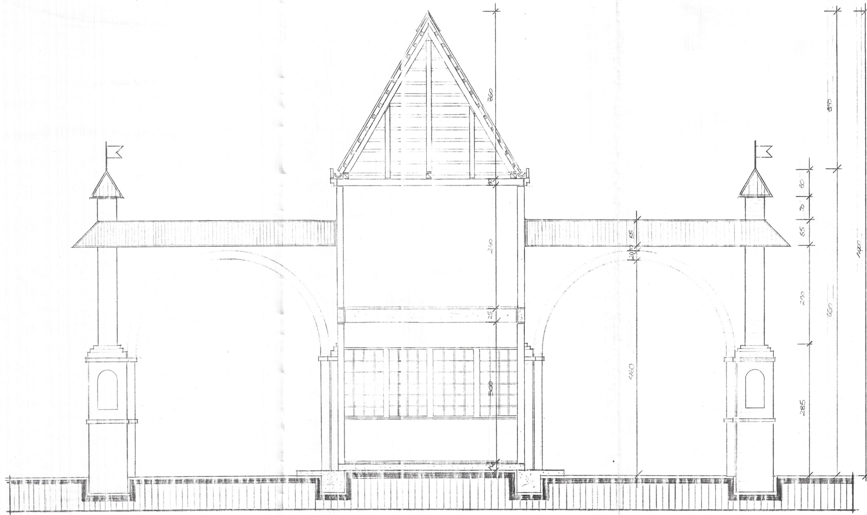
PORTAL COPIE A A' ESC. 1:50
