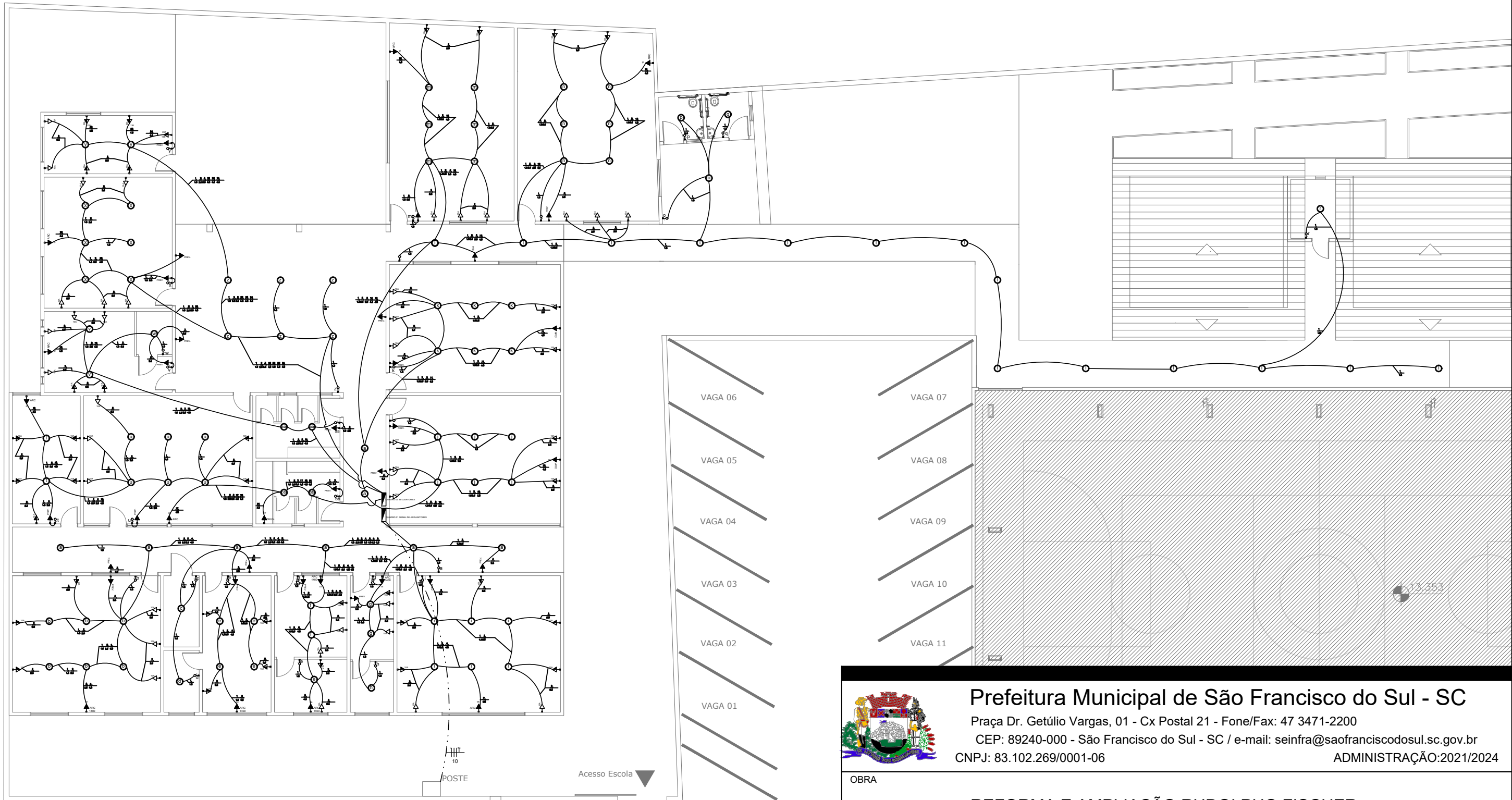
PLANTA BAIXA ELÉTRICA ESCALA 1/100
