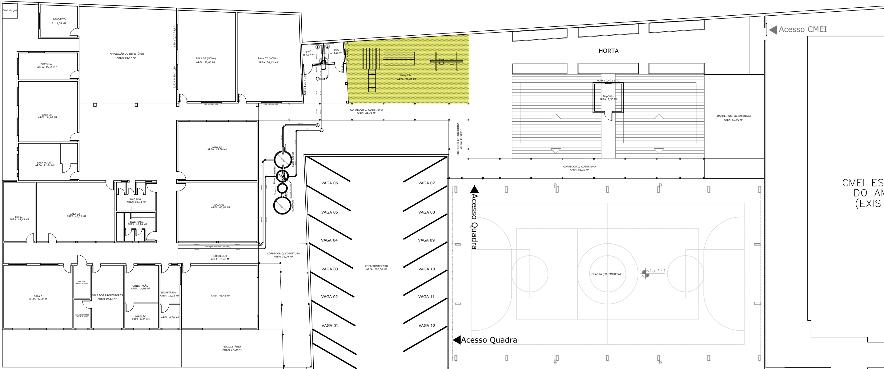
PLANTA BAIXA HIDROSSANITÁRIO ESCALA 1/100
