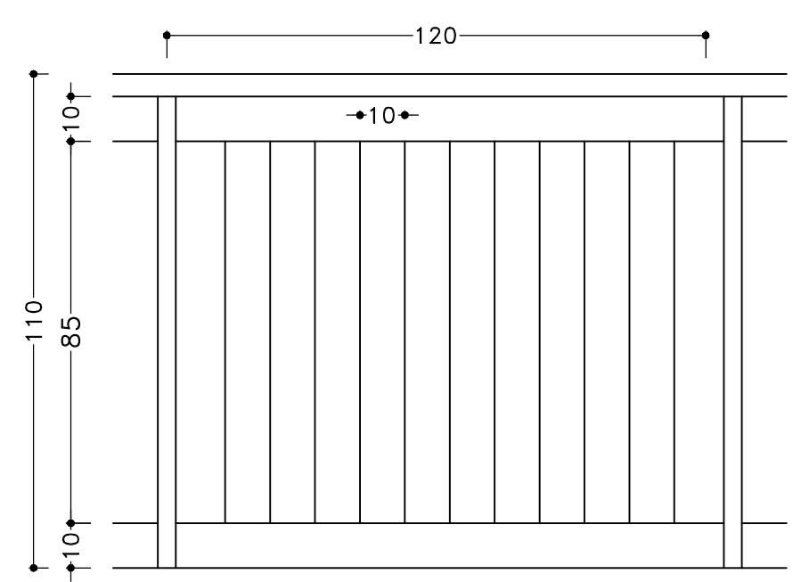
Detalher Guarda-Corpo Escala .....1/15
