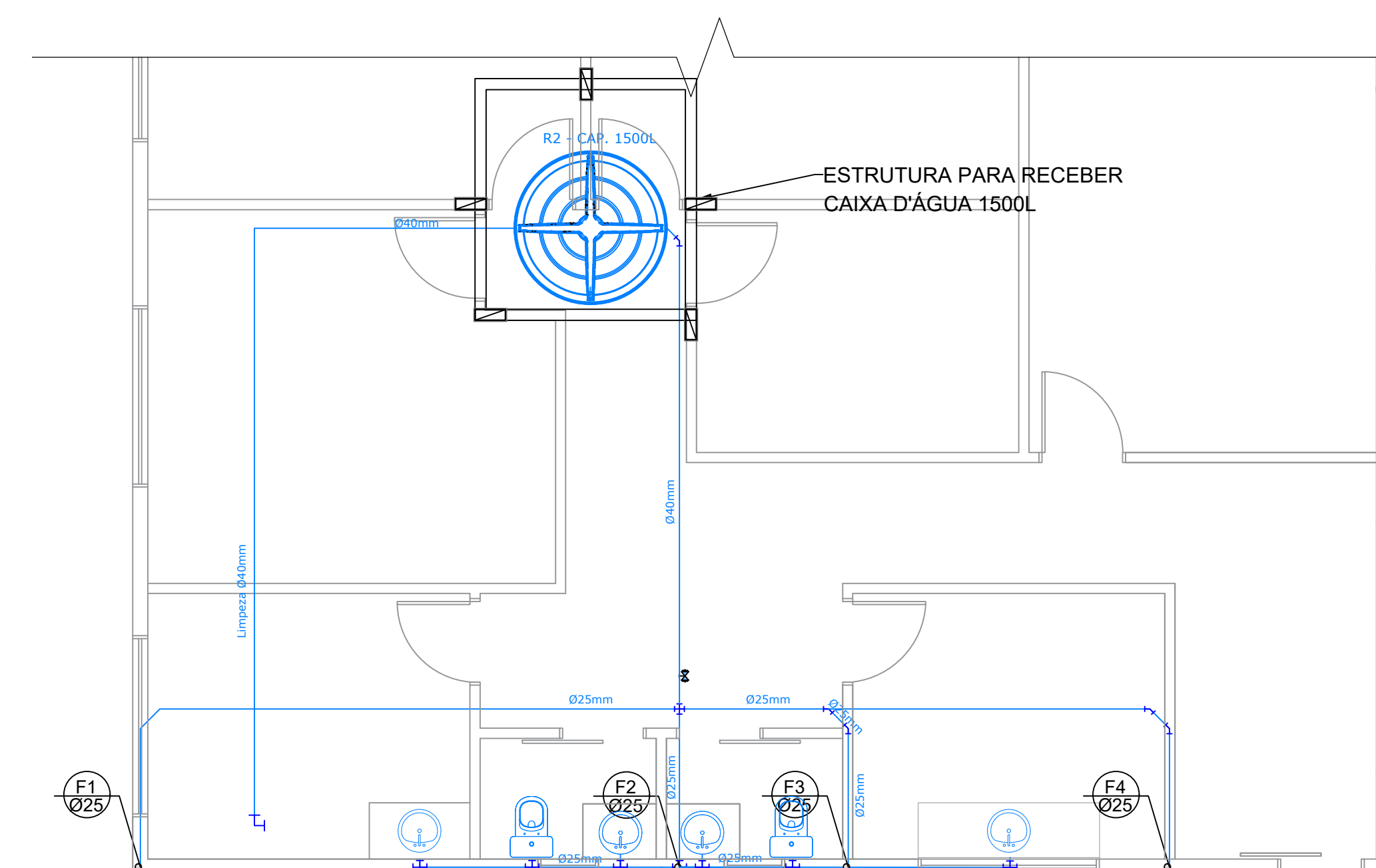
Detalhamento A.F. Escala .....1/50
