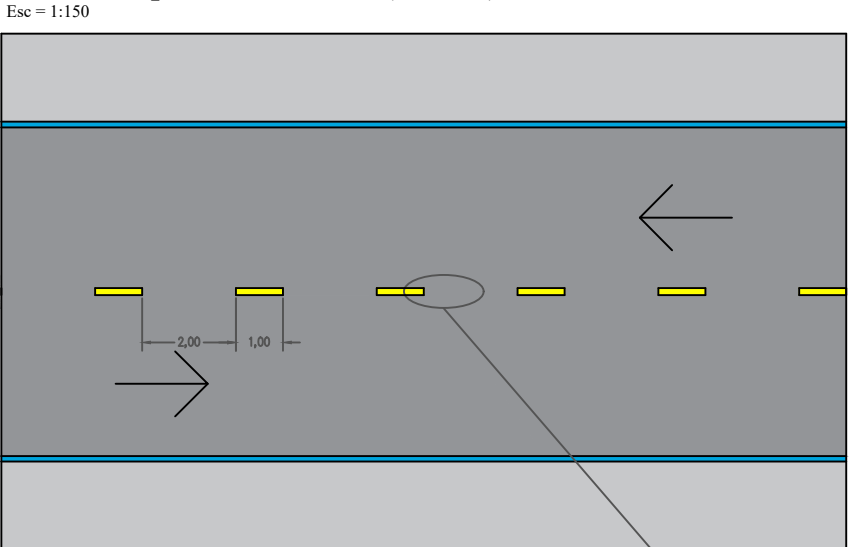
Linha Simples Seccionada (LFO-2)
