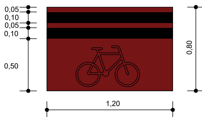
Detalhe da Pintura da Ciclorota S/E
