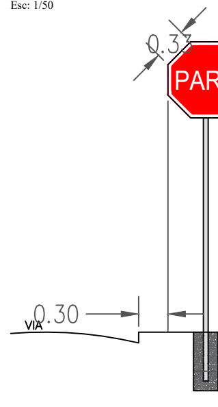
Detalhe Placa Regulamentação R1
