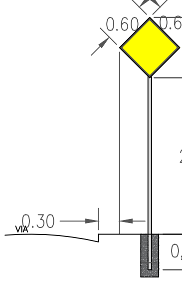
Detalhe Placa Advertência Lado de 60 cm
