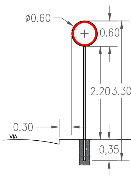
Detalhe Placa Regulamentação Diâmetro de 60 cm
